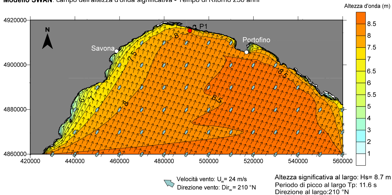
FIGURA 11-6 - RISULTATO DELLA PROPAGAZIONE DELLO STATO DI MARE OTTENUTO CON IL MODELLO SWAN. T_R=250 ANNI – DIREZIONE AL LARGO 210^\circ N
