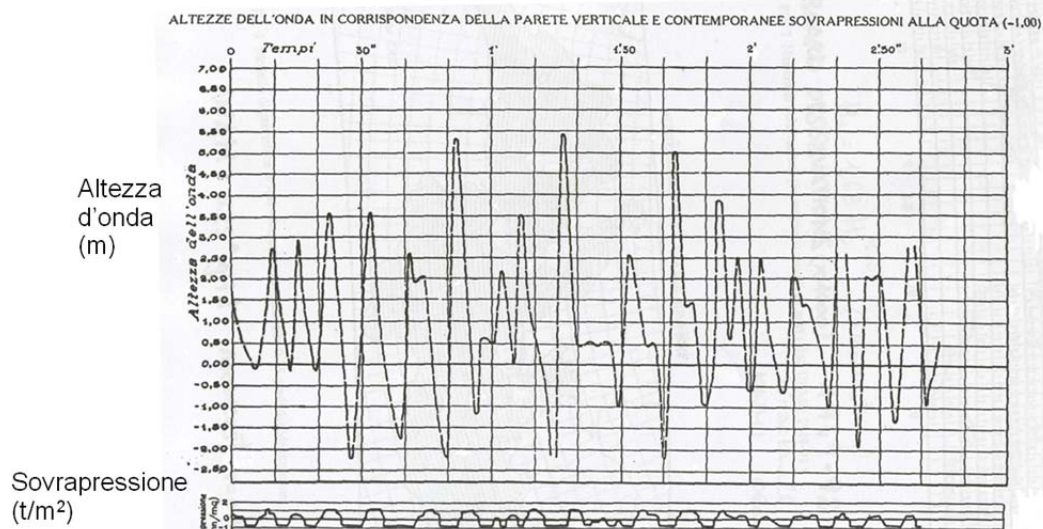
FIGURA 4-2. ESEMPIO DI REGISTRAZIONE ONDAMETRICA EFFETTUATA SUL CASSONE SPECIALE DELLA DIGA FORANEA DI GENOVA (FONTE: ANNALI DEI LAVORI PUBBLICI GIÀ GIORNALE DEL GENIO CIVILE - ANNO 1932)
