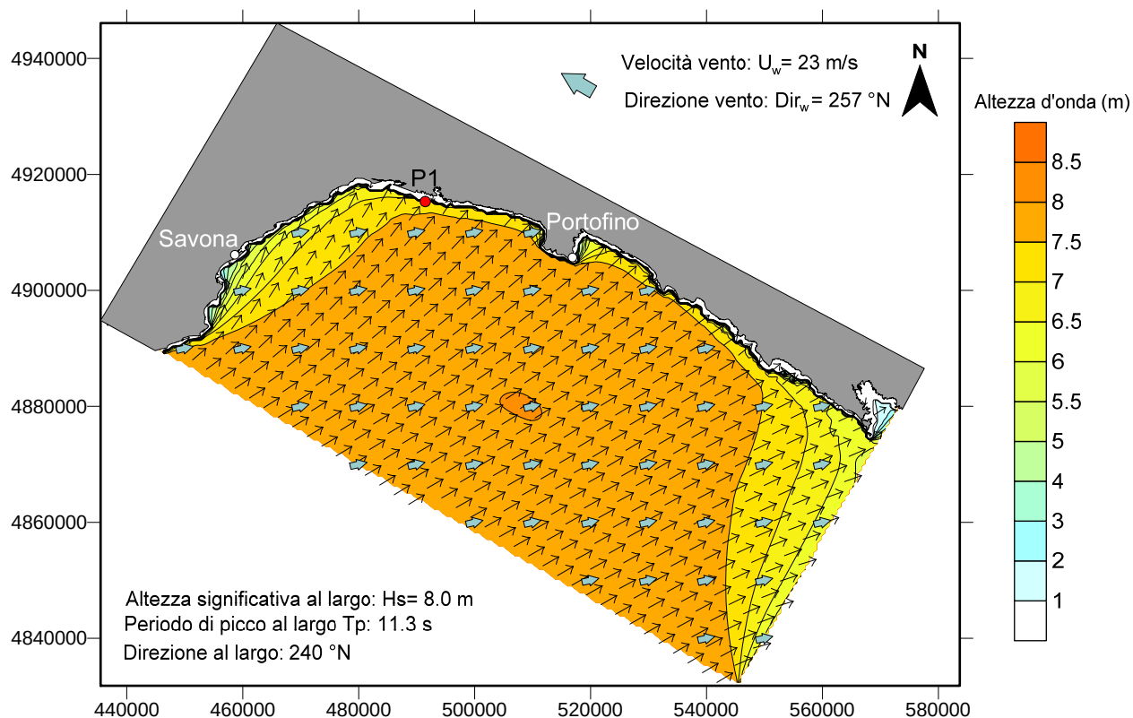
FIGURA 11-4 - RISULTATO DELLA PROPAGAZIONE DELLO STATO DI MARE OTTENUTO CON IL MODELLO SWAN. T_R = 100 ANNI DIREZIONE AL LARGO 240^\circ \text{N} .
