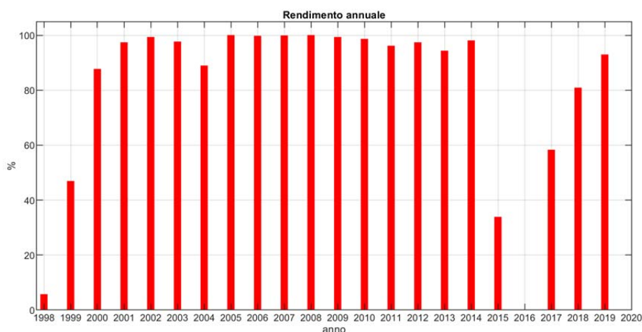
FIGURA 5-5. RENDIMENTO DELL'ANEMOMETRO INSTALLATO PRESSO LA STAZIONE MAREOGRAFICA RMN DI GENOVA (PERIODO DI RIFERIMENTO 1998-1999)
