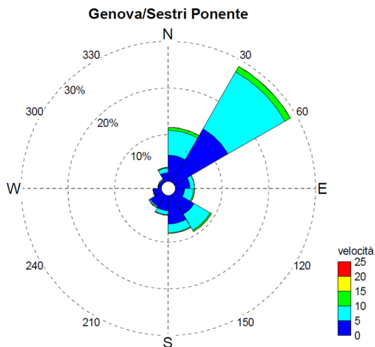
FIGURA 5-9. DISTRIBUZIONE DELLE VELOCITÀ DEL VENTO, IN METRI AL SECONDO, REGISTRATE DALLA STAZIONE METEOROLOGICA DI GENOVA-SESTRI DAL 1963 AL 2007. FONTE: "VENTO E PORTI - ANALISI STATISTICA DEI DATI STORICI DI VENTO REGISTRATI DALLE STAZIONI ANEMOMETRICHE".
