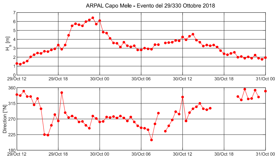
FIGURA 6-11. EVENTO METEO MARINO DEL 29-30 OTTOBRE 2018 REGISTRAZIONI DELLA BOA ONDAMETRICA ARPAL DI CAPO MELE.
