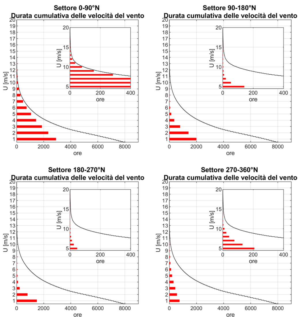
FIGURA 5-8. DURATA CUMULATIVA MEDIA DELLE VELOCITÀ DEL VENTO OSSERVATE PRESSO LA STAZIONE RMN DI GENOVA (GEN. 1999-NOV. 2019). LA CURVA NERA RAPPRESENTA LA DURATA CUMULATA COMPLESSIVA.
