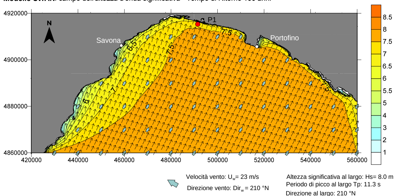
FIGURA 11-3 - RISULTATO DELLA PROPAGAZIONE DELLO STATO DI MARE OTTENUTO CON IL MODELLO SWAN. T_R = 100 ANNI DIREZIONE AL LARGO 210^\circ \text{N} .
