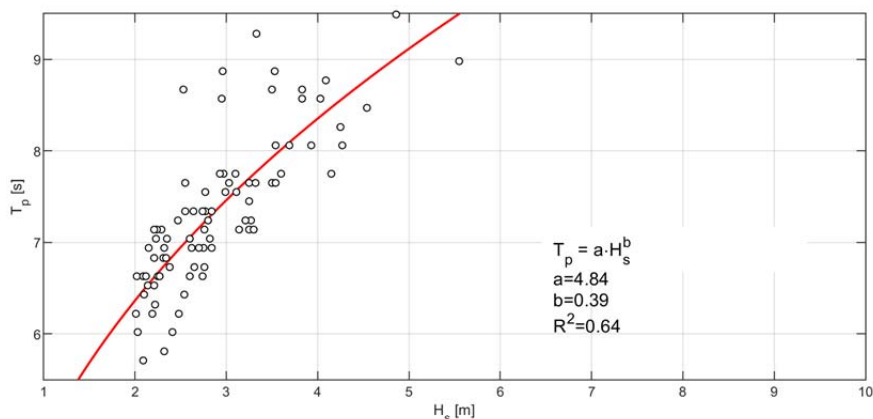
FIGURA 8-10. CORRELAZIONE PER I VALORI H_s - T_p AL COLMO DELLE MAREGGIATE PER IL SETTORE DI TRAVERSIA 105-180 °N
