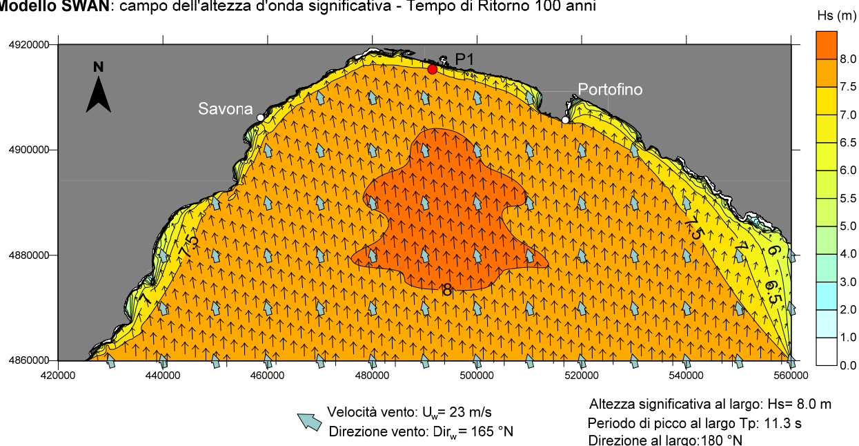
FIGURA 11-2 – RISULTATO DELLA PROPAGAZIONE DELLO STATO DI MARE OTTENUTO CON IL MODELLO SWAN. T_R=100 ANNI – DIREZIONE AL LARGO 180^\circ \text{N}
