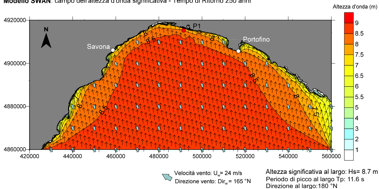
FIGURA 11-5 - RISULTATO DELLA PROPAGAZIONE DELLO STATO DI MARE OTTENUTO CON IL MODELLO SWAN. T_R = 250 ANNI – DIREZIONE AL LARGO 180^\circ \text{N}
