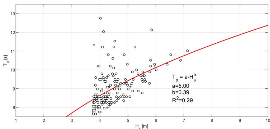
FIGURA 8-9. CORRELAZIONE PER I VALORI H_s - T_p AL COLMO DELLE MAREGGIATE PER IL SETTORE DI TRAVERSIA 180-240°N
