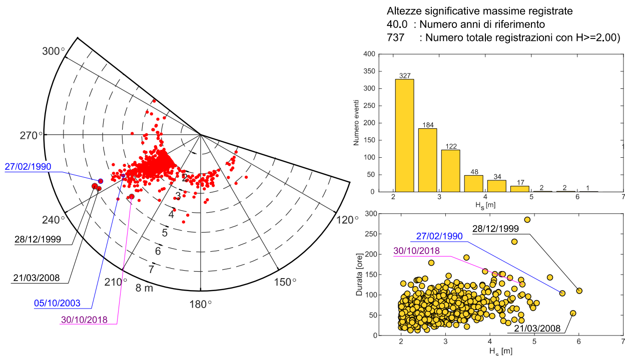
FIGURA 6-19. DISTRIBUZIONE DELLE ALTEZZE D'ONDA MASSIME ASSOCIATE AGLI EVENTI DI MAREGGIATA RICOSTRUITI DAL DICCA AL LARGO DI LA SPEZIA NEL PERIODO 1979-2018
