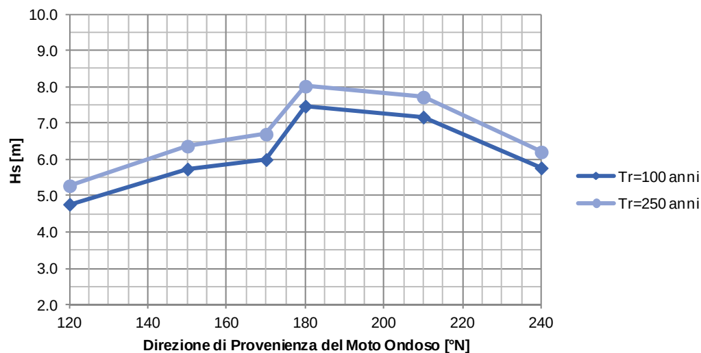
FIGURA 11-12 - ALTEZZA D'ONDA SIGNIFICATIVA OTTENUTA NEL PUNTO P1 IN FUNZIONE DELLA DIREZIONE DI PROVENIENZA AL LARGO PER GLI STATI DI MARE ESTREMI CON TEMPO DI RITORNO TR 100 ANNI E TR 250 ANNI.
