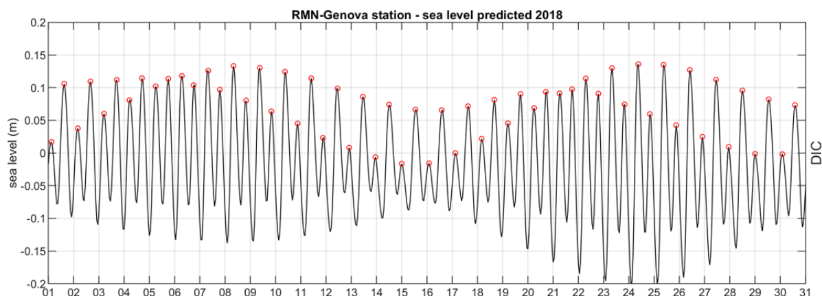
FIGURA 12-4. RICOSTRUZIONE DELLA MAREA ASTRONOMICA EFFETTUATA PER LA STAZIONE MAREOGRAFICA DI GENOVA PER IL MESE DI DICEMBRE 2018 APPLICANDO LE COSTANTI ARMONICHE OTTENUTE.
