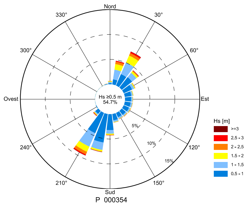
FIGURA 6-15. DISTRIBUZIONE DIREZIONALE DELL'ALTEZZA D'ONDA SIGNIFICATIVA H_s RICOSTRUITA DAL DICCA NEI PUNTI P_000354 E P_000391 AL LARGO DI CAPO MELE - PERIODO 1979-2018.
