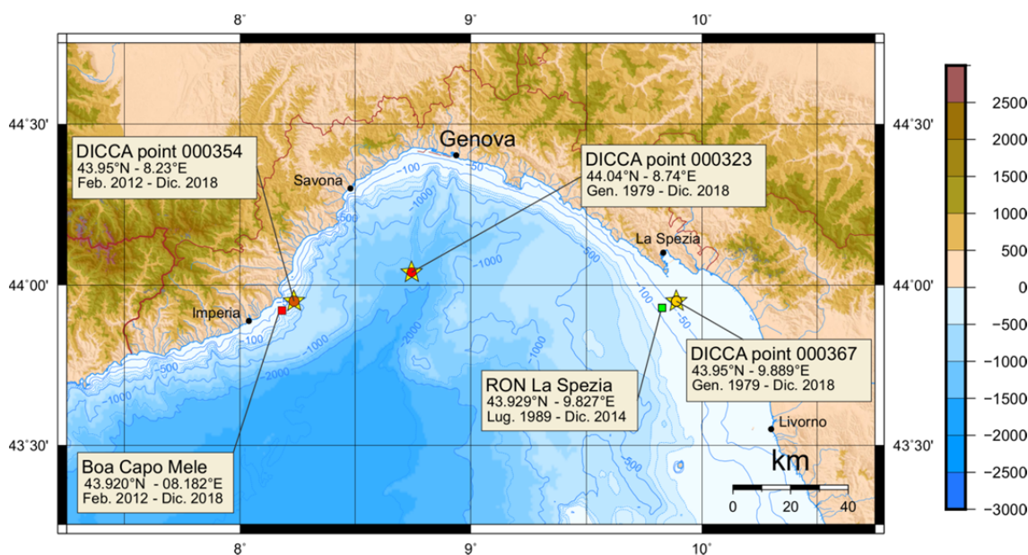
FIGURA 6-1. LOCALIZZAZIONE E DETTAGLI DELLE DIVERSE FONTI DI DATI DI MOTO ONDOSO UTILIZZATE PER LO STUDIO METEOMARINO
