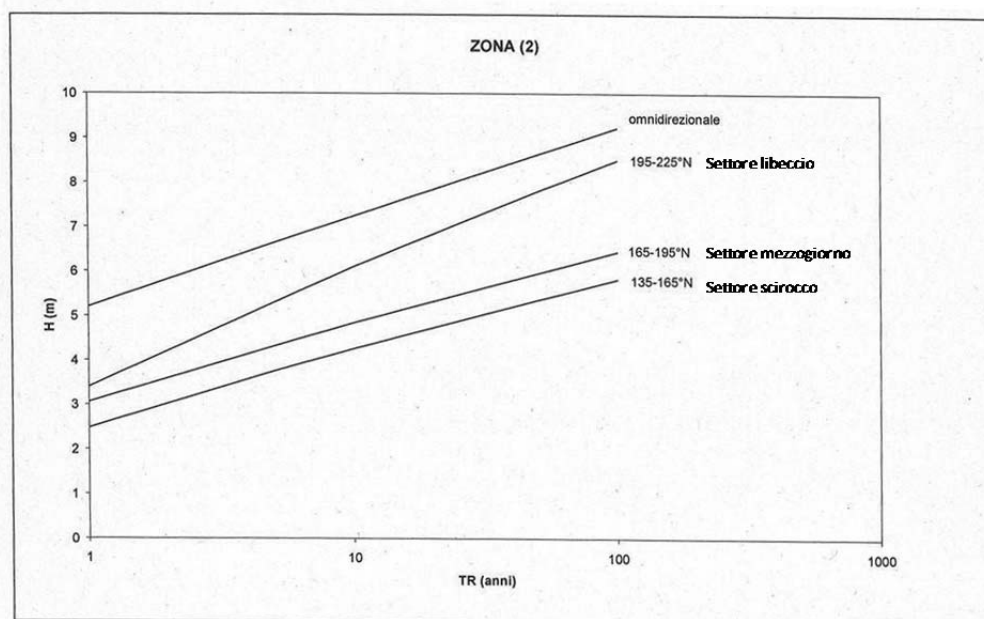
FIGURA 3-1. CORRELAZIONE H_s - T_R A LARGO DEL PORTO DI GENOVA (BOCCOTTI, 1986)
