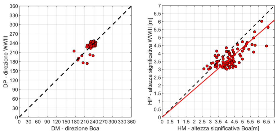
FIGURA 7-3. CONFRONTO ASINCRONO TRA I VALORI AL COLMO DELLE MAREGGIATE (CON H_s > 3.0 M) REGISTRATI DALLA BOA RON DI LA SPEZIA TRA IL 1989 ED IL 2014 E QUELLI RICOSTRUITI DAL DICCA CON IL MODELLO WWIII IN PROSSIMITÀ DELLA BOA.
