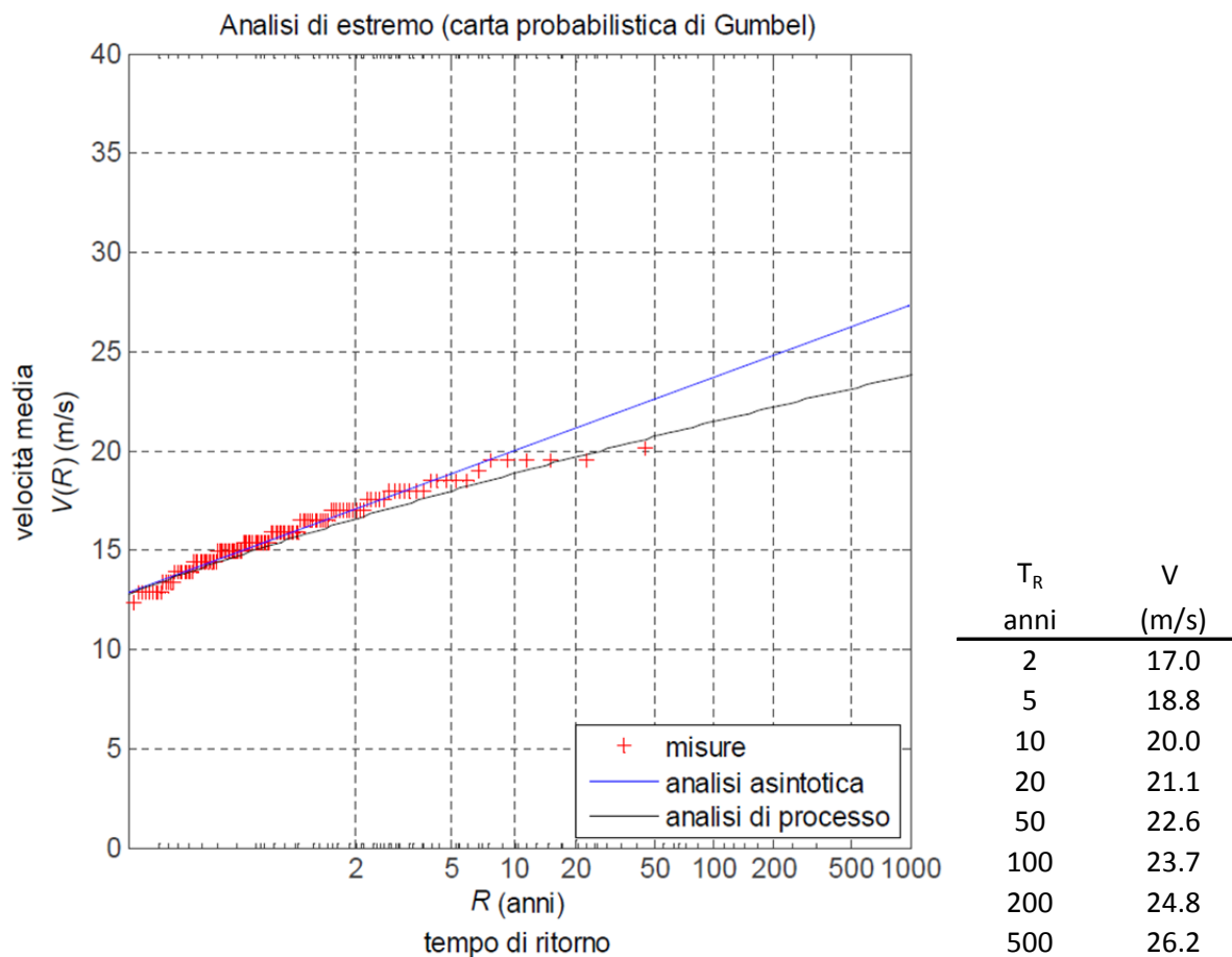
FIGURA 5-14. ADATTAMENTO DEI VALORI ESTREMI ANNUALI DI VENTO REGISTRATI DALLA STAZIONE METEO GENOVA-SESTRI (1963-2008) ALLA DISTRIBUZIONE DI PROBABILITÀ DEI VALORI ESTREMI TIPO I DI GUMBEL. ESTRATTO DA "VENTO E PORTI - ANALISI STATISTICA DEI DATI STORICI DI VENTO REGISTRATI DALLE STAZIONI ANEMOMETRICHE".
