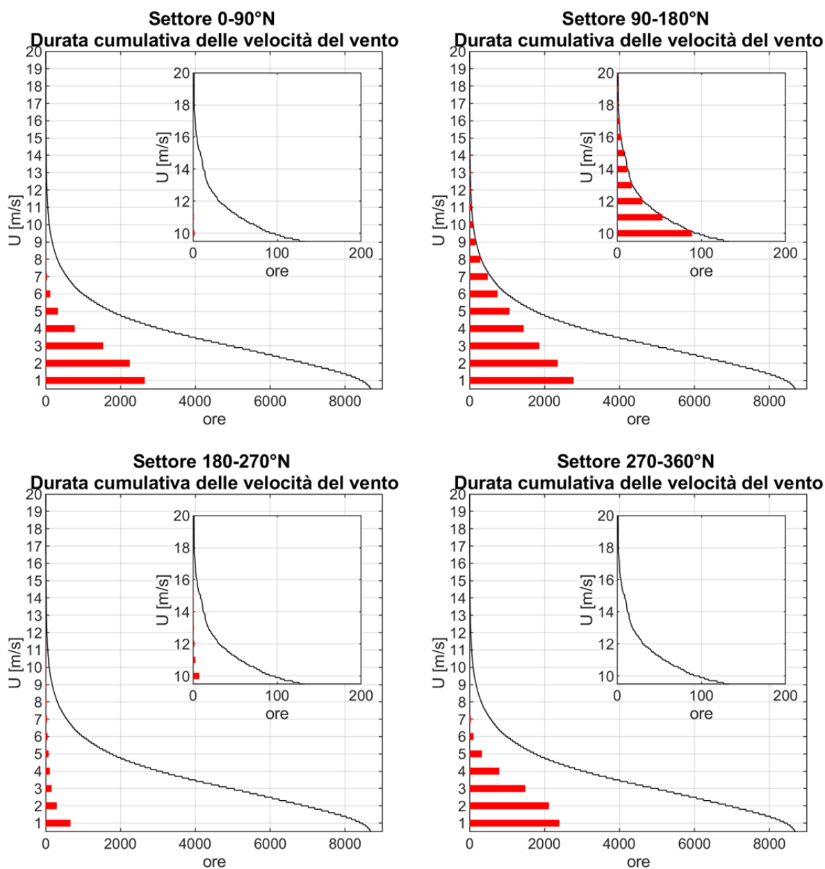
FIGURA 5-13. DURATA CUMULATIVA DELLE VELOCITÀ DEL VENTO OSSERVATE PRESSO LA STAZIONE ARPAL DI PUNTA VAGNO (2015-2019). LA CURVA NERA RAPPRESENTA LA DURATA CUMULATA COMPLESSIVA.
