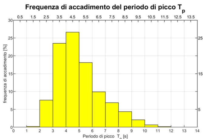
FIGURA 9-5. FREQUENZA DI ACCADIMENTO DEL PERIODO DI PICCO T_p .
