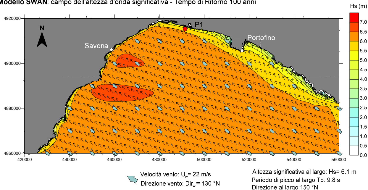
FIGURA 11-8 - RISULTATO DELLA PROPAGAZIONE DELLO STATO DI MARE OTTENUTO CON IL MODELLO SWAN. T_R=100 ANNI – DIREZIONE AL LARGO 150^\circ N
