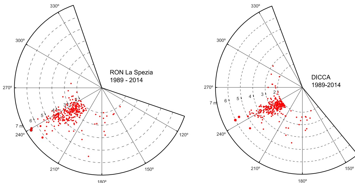
FIGURA 7-2. DISTRIBUZIONE DEI VALORI DI ALTEZZA D'ONDA H_s AL COLMO DELLE MAREGGIATE REGISTRATE DALLA BOA RON DI LA SPEZIA (SINISTRA) E RICOSTRUITE DAL DICCA (DESTRA) NEL PERIODO 1989 - 2014.
