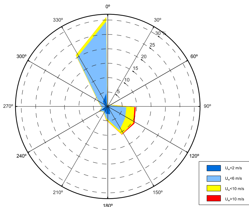
FIGURA 5-12. DISTRIBUZIONE DEI VENTI MISURATI DALLA STAZIONE METEOROLOGICA ARPAL DI PUNTA VAGNO. PERIODO DI RIFERIMENTO 2015-2019.
