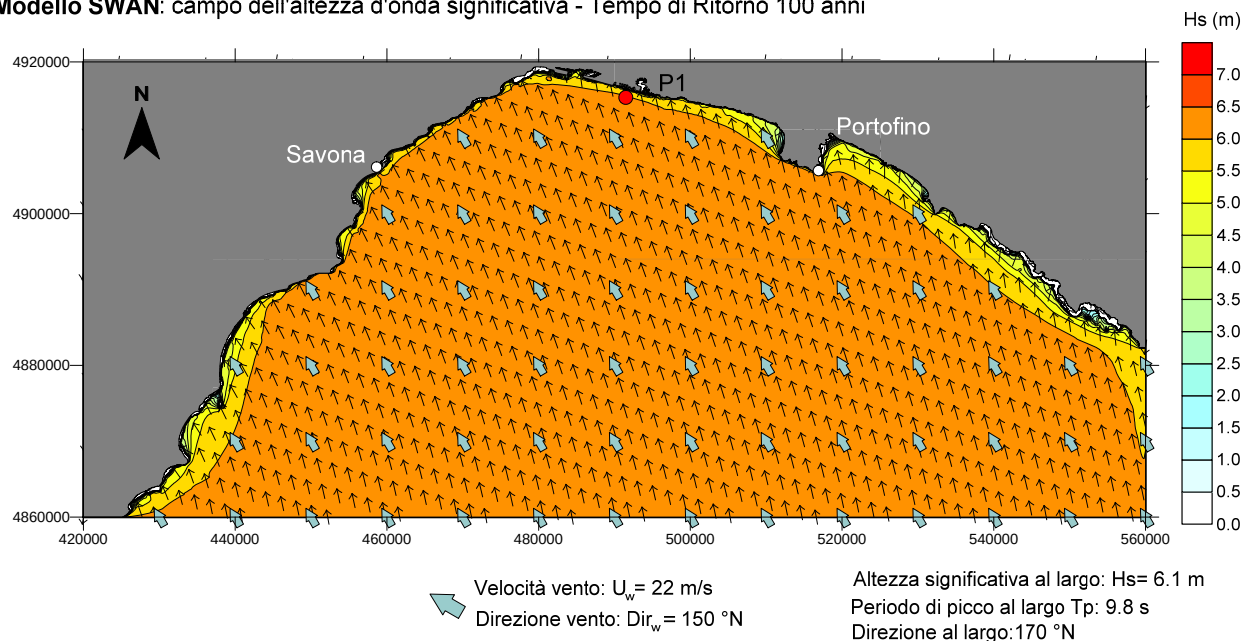
FIGURA 11-9 - RISULTATO DELLA PROPAGAZIONE DELLO STATO DI MARE OTTENUTO CON IL MODELLO SWAN. T_R=100 ANNI – DIREZIONE AL LARGO 170^\circ N
