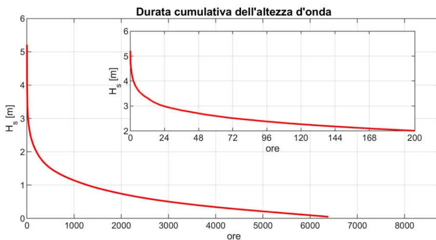
FIGURA 10-3. DURATA CUMULATIVA SU BASE ANNUALE DELL'ALTEZZA D'ONDA NEL PUNTO SOTTOCOSTA P1.
