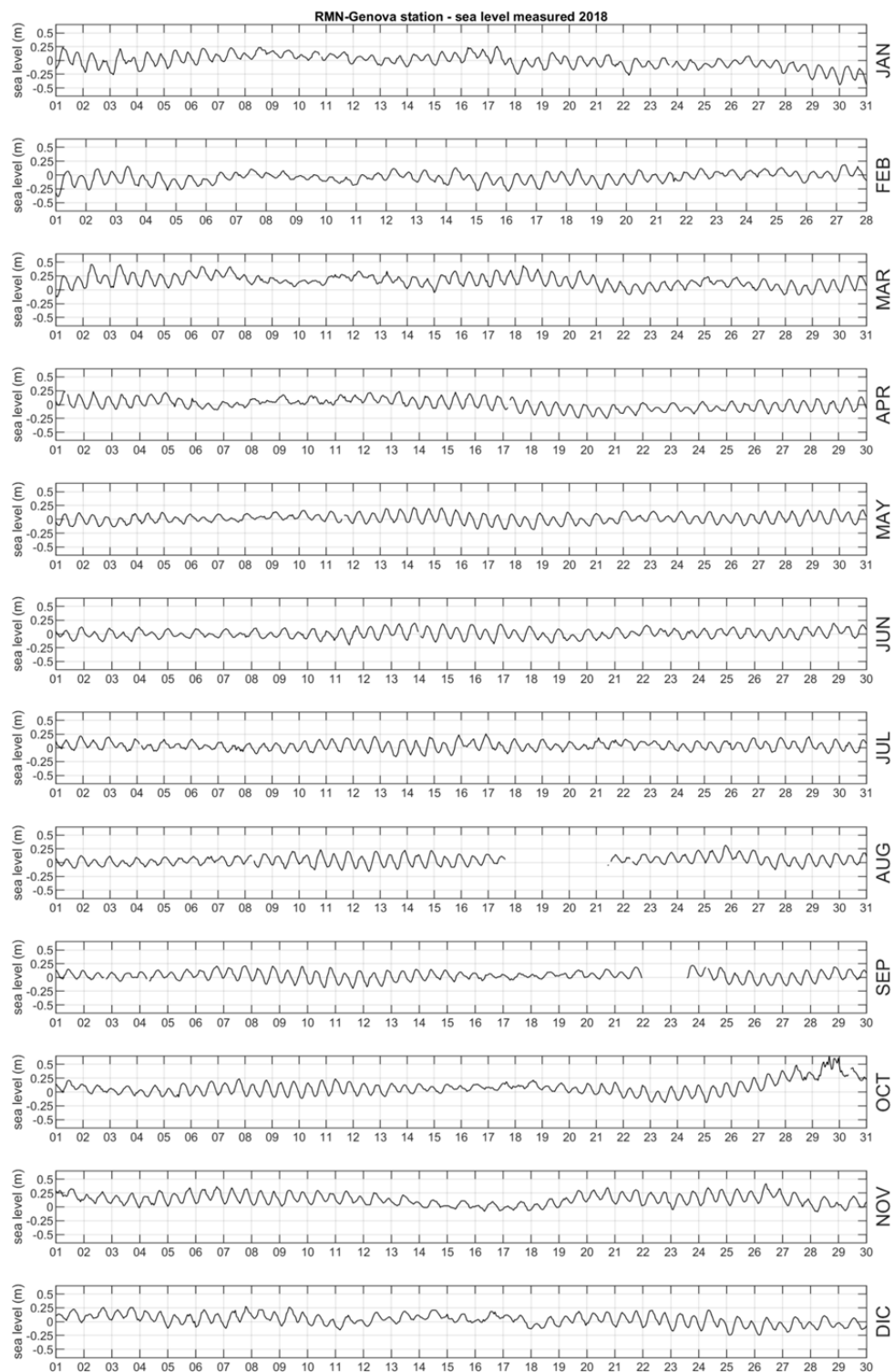
FIGURA 12-2. MISURE DI LIVELLO EFFETTUATE NELL'ANNO 2018 DALLA STAZIONE RMN DI GENOVA.
