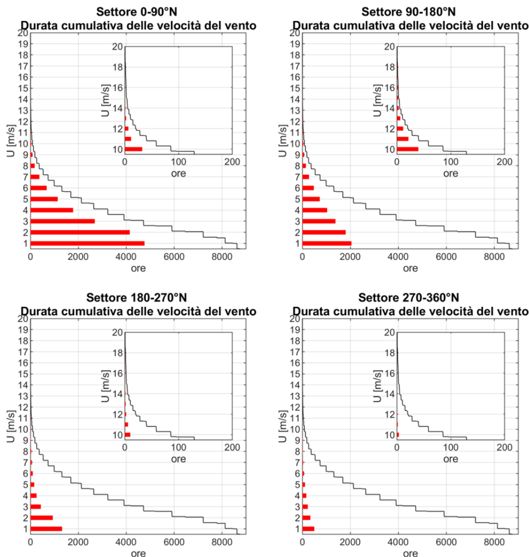
FIGURA 5-11. DURATA CUMULATIVA DELLE VELOCITÀ DEL VENTO OSSERVATE PRESSO LA STAZIONE DI GENOVA SESTRI (GEN 2008-DIC 2019). LA CURVA NERA RAPPRESENTA LA DURATA CUMULATA COMPLESSIVA.
