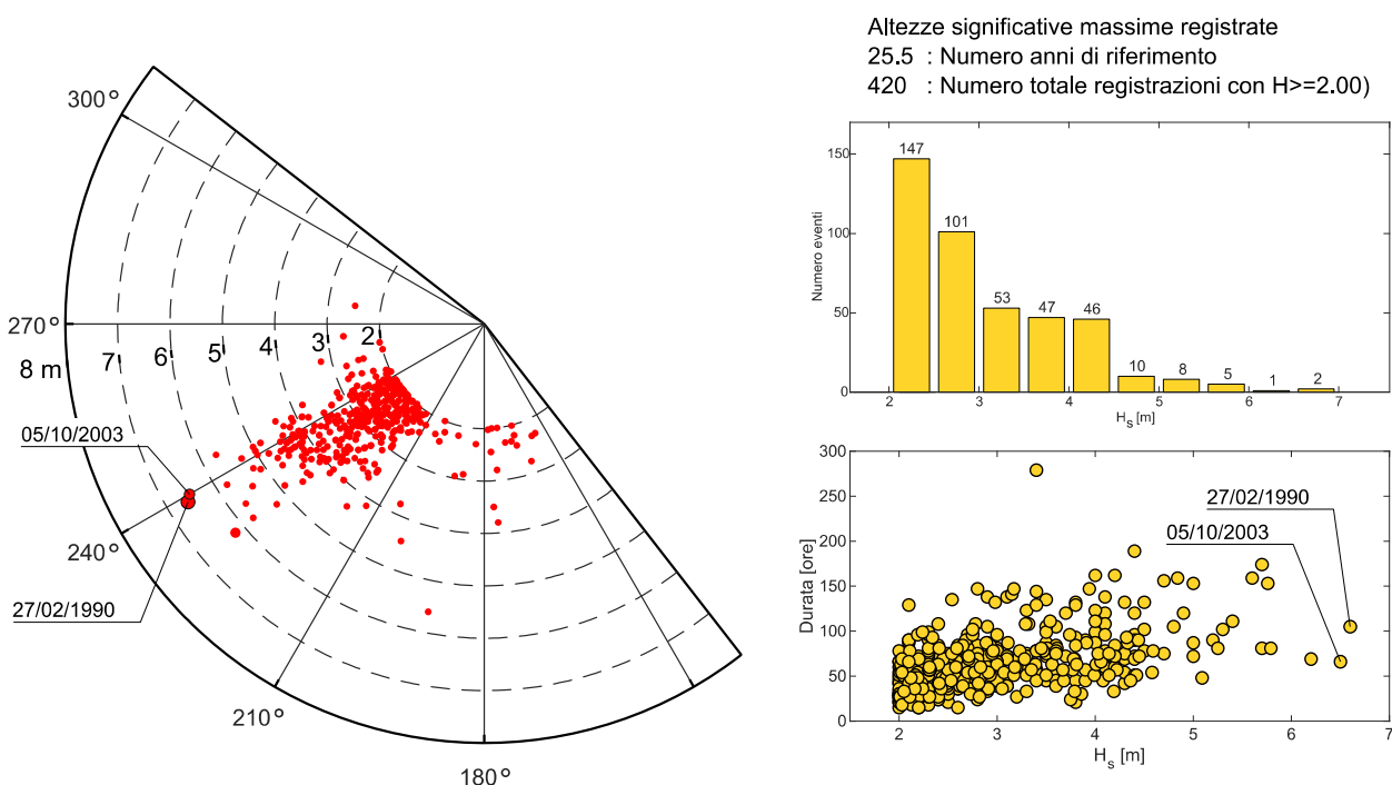
FIGURA 6-5. DISTRIBUZIONE DELLE ALTEZZE D'ONDA MASSIME ASSOCIATE AGLI EVENTI DI MAREGGIATA OSSERVATI DALLA BOA RON DI LA SPEZIA NEL PERIODO 1989-2014.
