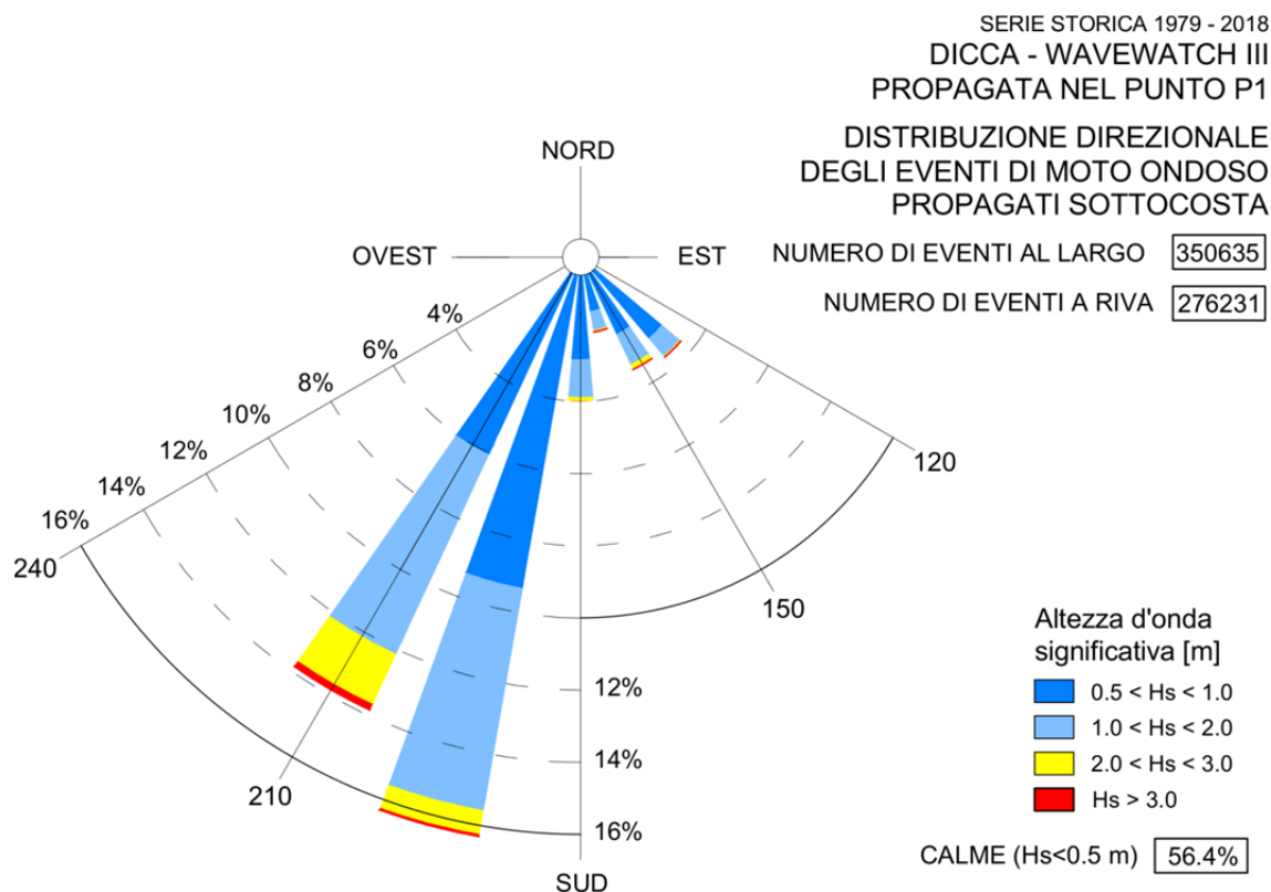
FIGURA 10-2. DISTRIBUZIONE DIREZIONALE DEGLI EVENTI DI MOTO ONDOSO PROPAGATI SOTTOCOSTA NEL PUNTO P1 CON IL MODELLO DI INVERSA SPETTRALE
