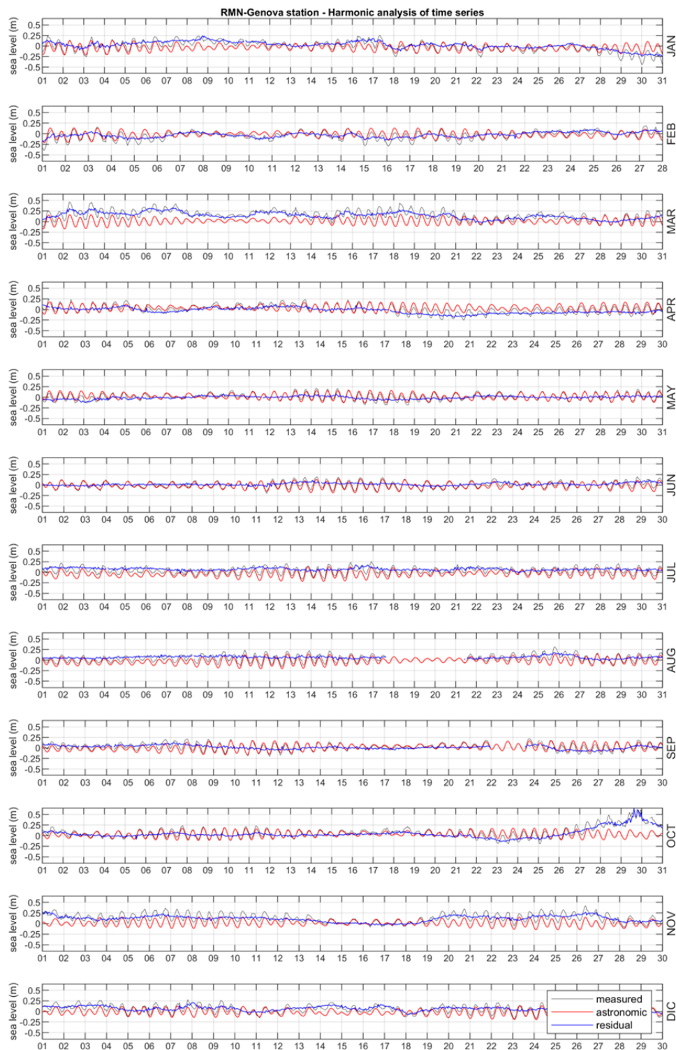
FIGURA 12-3. RICOSTRUZIONE DELLA MAREA ASTRONOMICA (IN ROSSO) E VALORI RESIDUI (IN BLU) SULLA BASE DEI LIVELLI MISURATI (IN NERO) DALLA STAZIONE RMN DI GENOVA PER L'ANNO 2018
