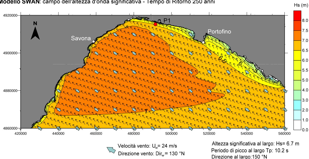
FIGURA 11-10 – RISULTATO DELLA PROPAGAZIONE DELLO STATO DI MARE OTTENUTO CON IL MODELLO SWAN. Tr=250 ANNI – DIREZIONE AL LARGO 150^\circ N
