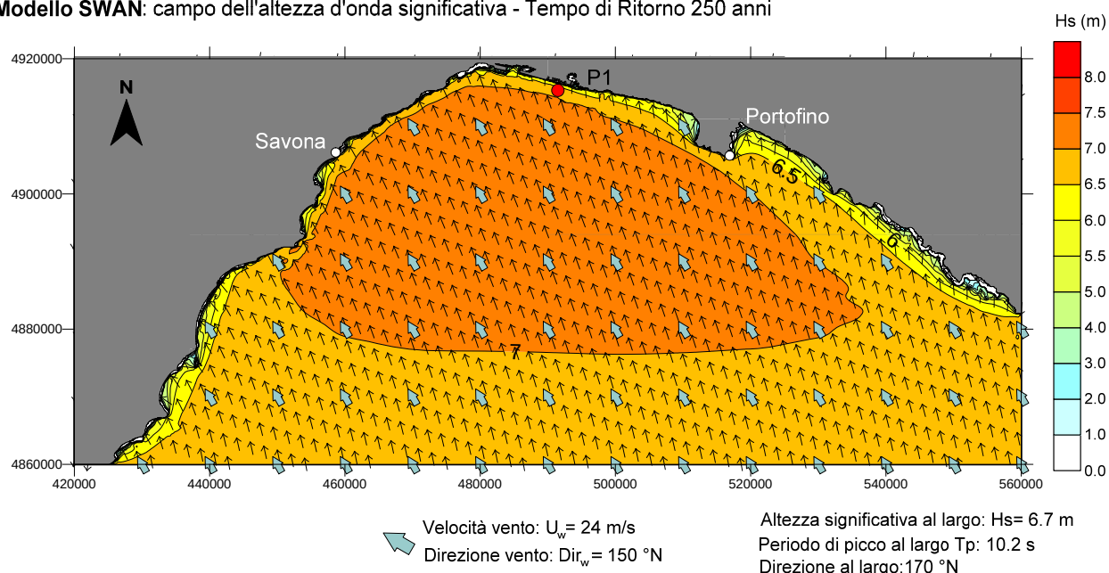
FIGURA 11-11 - RISULTATO DELLA PROPAGAZIONE DELLO STATO DI MARE OTTENUTO CON IL MODELLO SWAN. Tr=250 ANNI – DIREZIONE 170^\circ N
