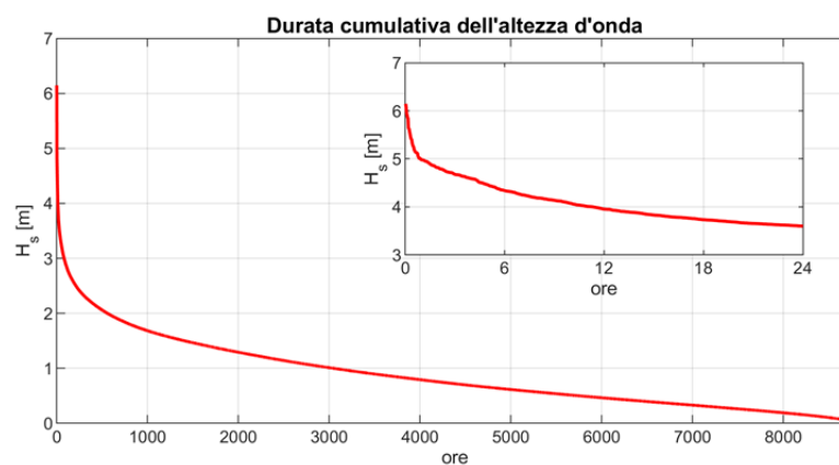
FIGURA 9-3. DURATA CUMULATIVA DEGLI EVENTI DI MOTO ONDOSO AL LARGO IN FUNZIONE DELL'ALTEZZA D'ONDA SIGNIFICATIVA H_s .
