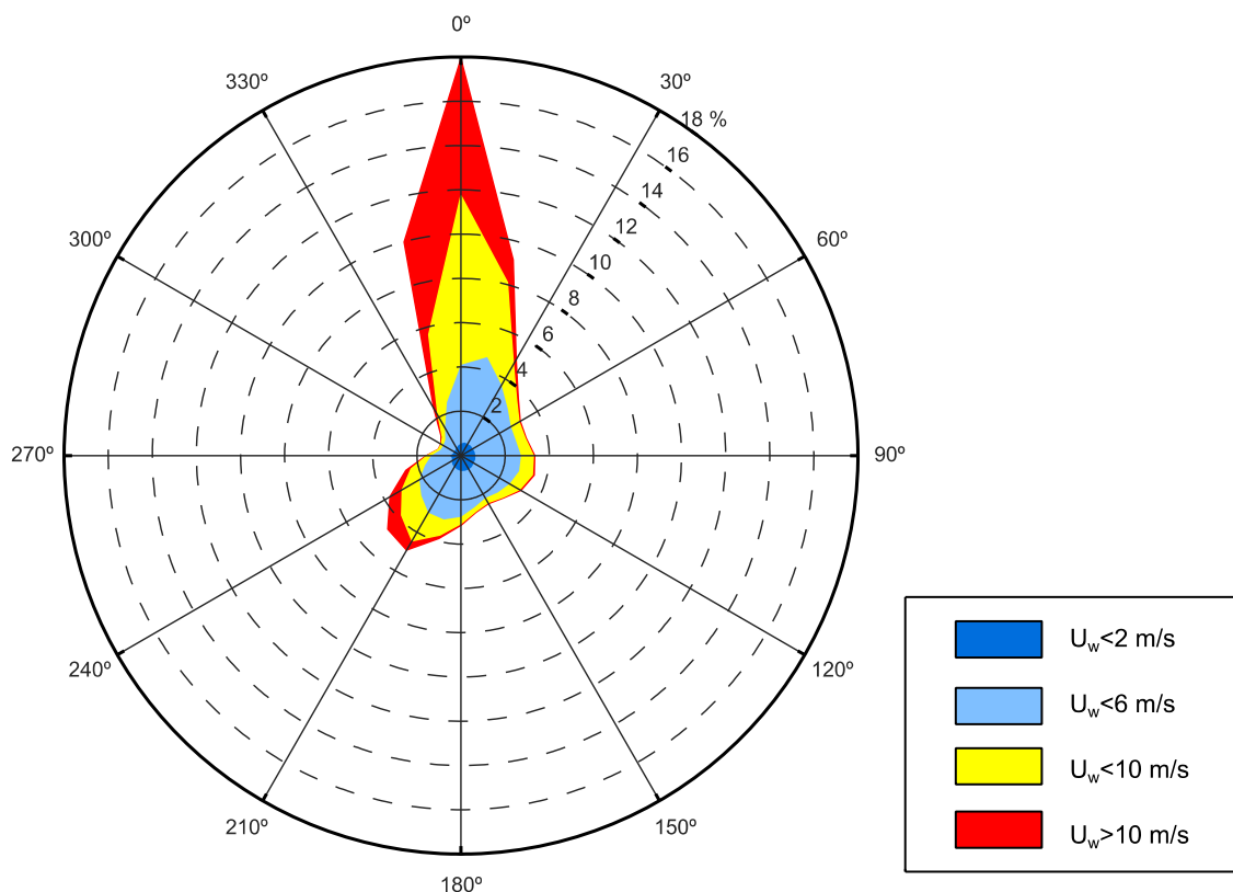
FIGURA 5-2. DISTRIBUZIONE DIREZIONALE DEI VENTI RICOSTRUITI DAL DICCA AL LARGO DEL GOLFO DI GENOVA NEL PUNTO 000323 DI COORDINATE 44.04°N - 8.74°E (PERIODO DI RIFERIMENTO 1979-2018)
