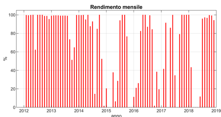
FIGURA 6-8. RENDIMENTO MENSILE DELLA BOA ONDAMETRICA DI CAPO MELE FEBBRAIO 2012 - DICEMBRE 2018.
