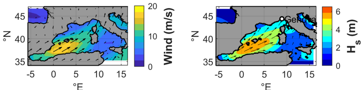
FIGURA A-2. CAMPI DI VENTO E DI ALTEZZA D'ONDA SIGNIFICATIVA H_s OTTENUTI A SEGUITO DELLA SIMULAZIONE CON IL MODELLO SWAN PER IL GIORNO 17 FEBBRAIO 1955
