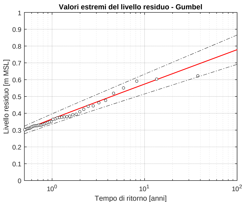
FIGURA 12-5. ANALISI STATISTICA DEI VALORI MASSIMI MENSILI DI LIVELLO RESIDUO (BLOCK MAXIMA) OSSERVATI ALLA STAZIONE MAREOGRAFICA RMN DI GENOVA (PERIODO DI RIFERIMENTO 1998-2018).
