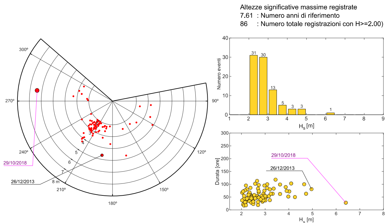
FIGURA 6-10. DISTRIBUZIONE DELLE ALTEZZE D'ONDA MASSIME ASSOCIATE AGLI EVENTI DI MAREGGIATA OSSERVATI DALLA BOA DI CAPO MELE PERIODO 2012-2018.
