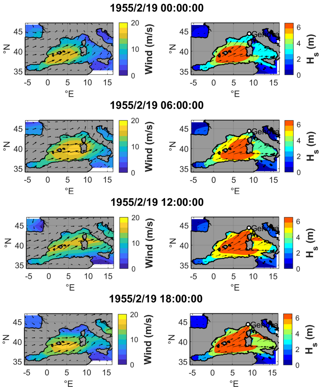
FIGURA A-4. CAMPI DI VENTO E DI ALTEZZA D'ONDA SIGNIFICATIVA H_s OTTENUTI A SEGUITO DELLA SIMULAZIONE CON IL MODELLO SWAN PER IL GIORNO 19 FEBBRAIO 1955
