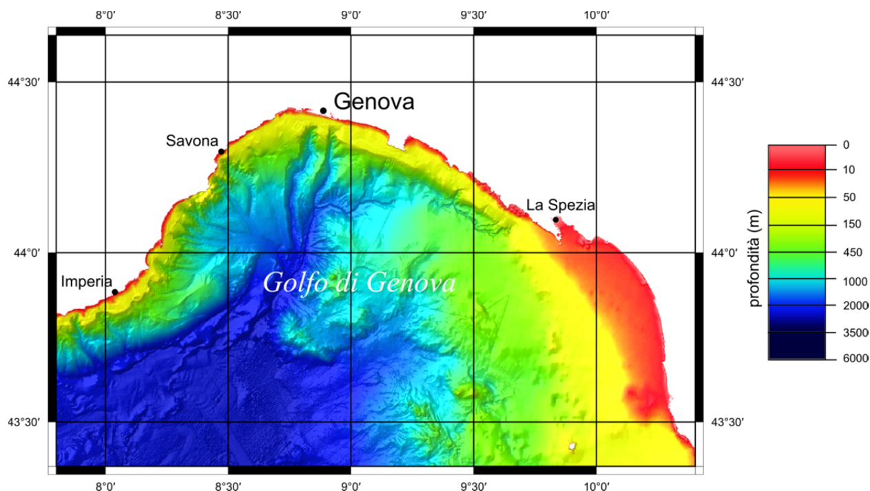
FIGURA 2-3. BATIMETRIA DEL GOLFO DI GENOVA
