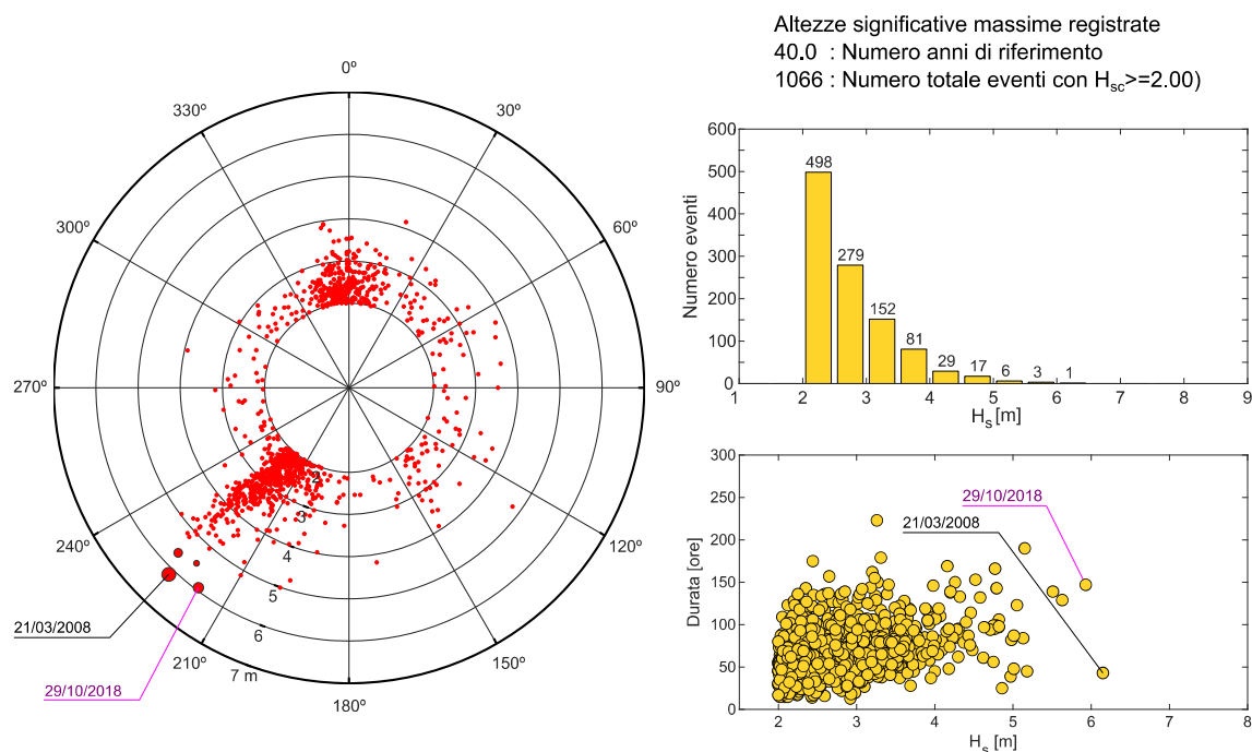
FIGURA 6-13. DISTRIBUZIONE DELLE ALTEZZE D'ONDA AL COLMO DELLE MAREGGIATE RICOSTRUITE AL LARGO DEL GOLFO DI GENOVA DAL DICCA NEL PUNTO 000323 PERIODO 1978 - 2018.
