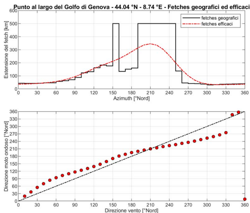
FIGURA 2-6. ESTENSIONE DEI FETCHES E LEGGE DI DEVIAZIONE VENTO/MARE AL LARGO DI GENOVA NEL PUNTO DI COORDINATE 44.04°N - 8.74°E.
