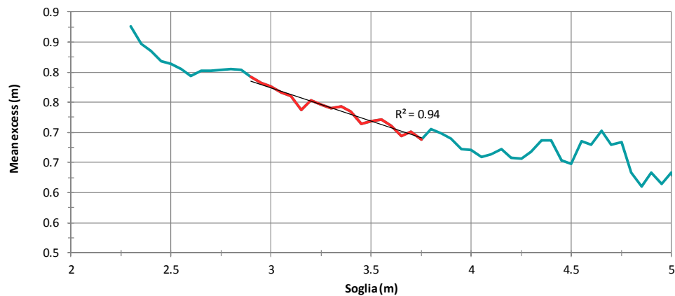
FIGURA 8-3 - MEAN RESIDUAL LIFE PLOT - SETTORE A: 180 - 240°N
