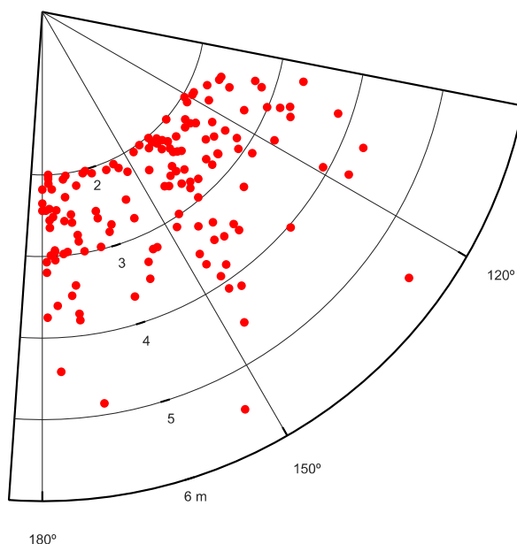
FIGURA 8-2. GENOVA LARGO DATI CALIBRATI - VALORI MASSIMI DI H_s OSSERVATI ALL'INTERNO DEL SETTORE DI TRAVERSIA 105-180 °N DURANTE LE MAREGGIATE RICOSTRUITE NEL PERIODO 1979-2018
