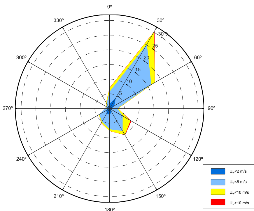
FIGURA 5-10. DISTRIBUZIONE DIREZIONALE DEI DATI VENTO SYNOP PER LA STAZIONE DI GENOVA-SESTRI PERIODO DI RIFERIMENTO GEN 2008-DIC 2019.
