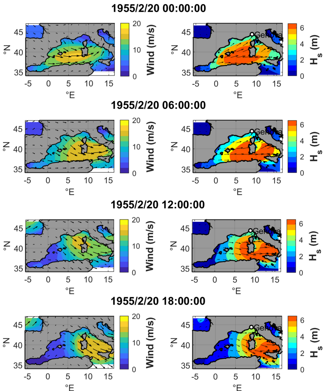
FIGURA A-5. CAMPI DI VENTO E DI ALTEZZA D'ONDA SIGNIFICATIVA H_s OTTENUTI A SEGUITO DELLA SIMULAZIONE CON IL MODELLO SWAN PER IL GIORNO 20 FEBBRAIO 1955
