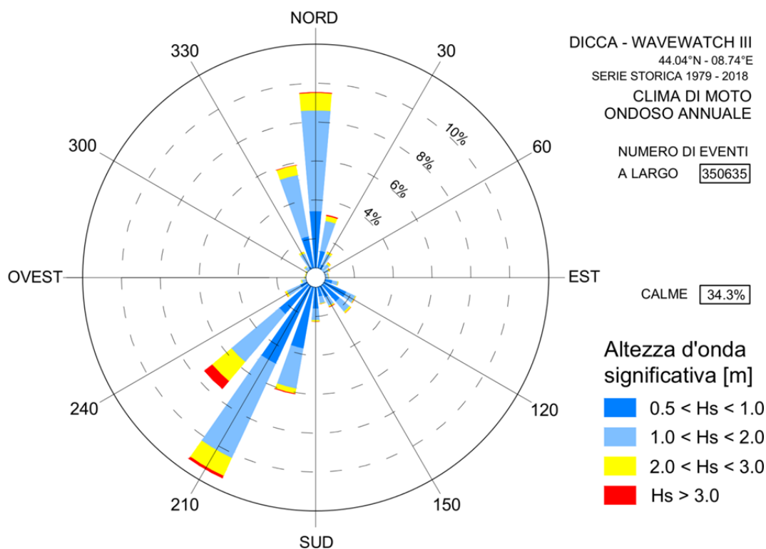
FIGURA 9-2. DISTRIBUZIONE DIREZIONALE DEGLI EVENTI DI MOTO ONDOSO RICOSTRUITI DAL DICCA AL LARGO DI GENOVA. PERIODO DI RIFERIMENTO (1979-2018)
