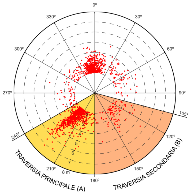
FIGURA 8-1 - GENOVA LARGO DATI CALIBRATI - DISTRIBUZIONE DIREZIONALE DEI VALORI DI H_s AL COLMO DELLE MAREGGIATE RICOSTRUIE NEL PERIODO 1979-2018
