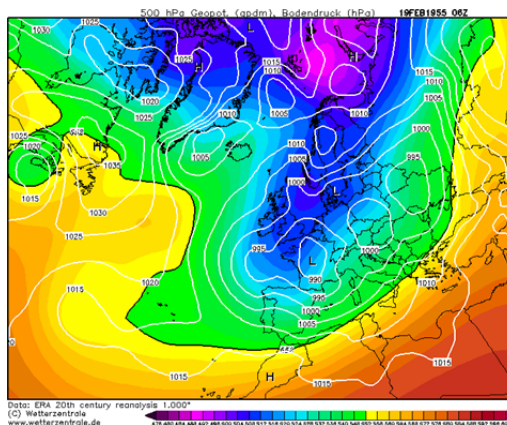
FIGURA A-1. ALTEZZA GEOPOTENZIALE IN REANALISI FORNITA DAL CENTRO METEOROLOGICO EUROPEO ECMWF PER IL 19 FEBBRAIO 1955 ALLE ORE 6:00
