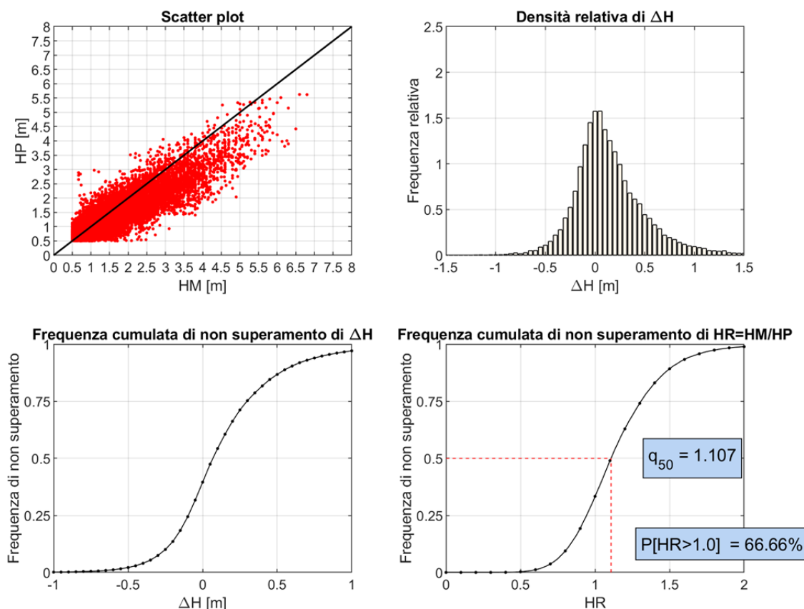
FIGURA 7-1. CONFRONTO DEI DATI DI MOTO ONDOSO RICOSTRUITI DAL DICCA (HP) UTILIZZANDO I DATI SINCRONI REGISTRATI DALLA BOA ONDAMETRICA RON DI LA SPEZIA (HM) NEL PERIODO 1989-2014.
