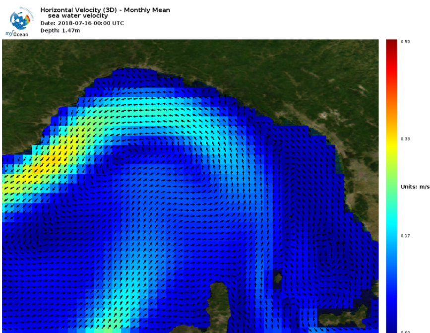
FIGURA 13-3. VALORE MEDIO DELLA CORRENTE SUPERFICIALE RICOSTRUITA PER IL MESE DI LUGLIO 2018.
