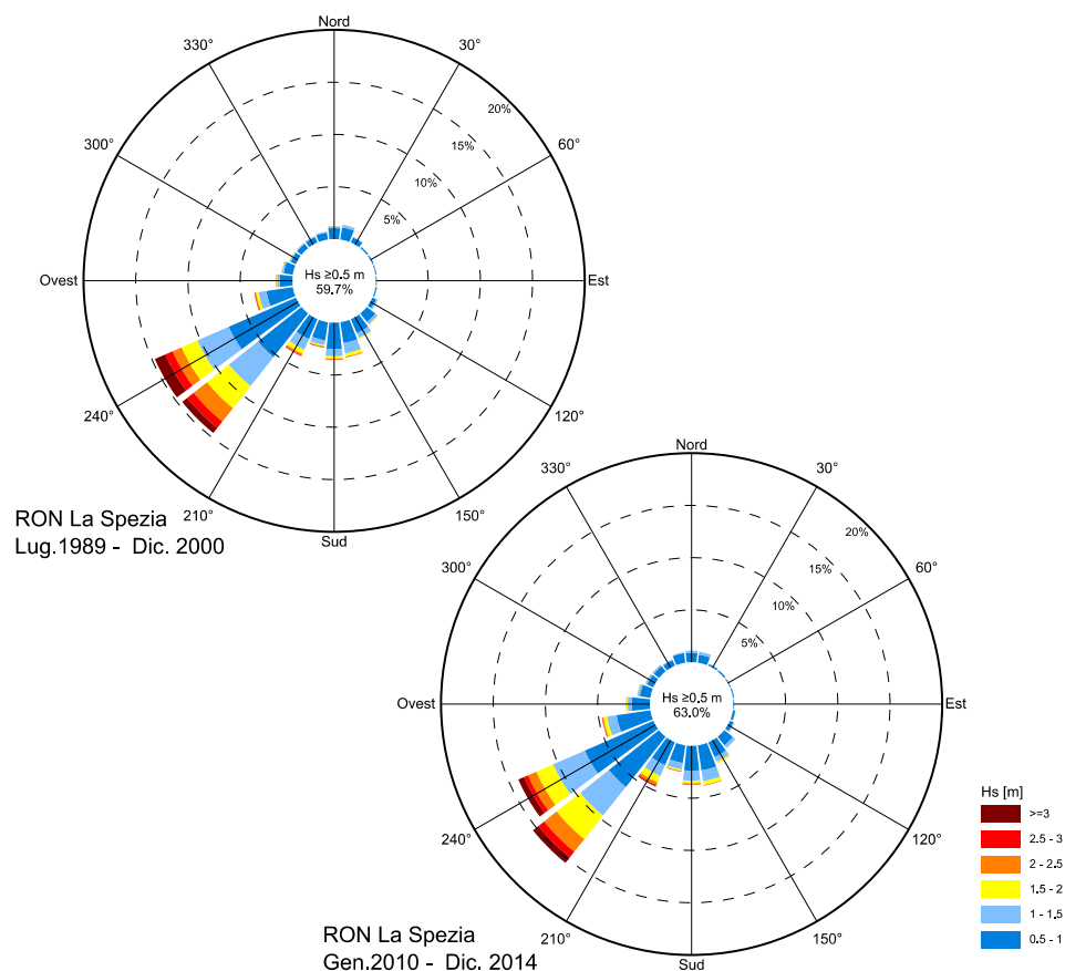
FIGURA 6-4. DISTRIBUZIONE DIREZIONALE DELL'ALTEZZA D'ONDA SIGNIFICATIVA H_s REGISTRATA DALLA BOA RON DI LA SPEZIA NEL PERIODO 1989-2000 E NEL PERIODO 2010-2014.
