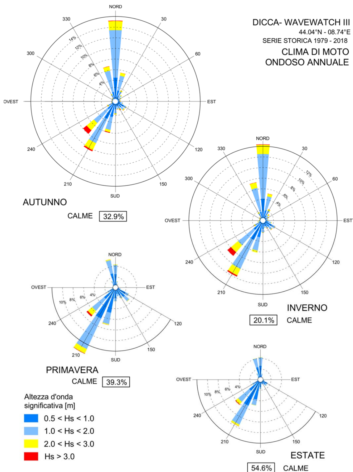
FIGURA 9-4. DISTRIBUZIONE DIREZIONALE DELL'ALTEZZA D'ONDA SIGNIFICATIVA H_s NEL PUNTO DI RICOSTRUZIONE DICCA 000323AL LARGO DI GENOVA SU BASE STAGIONALE (PERIODO DI RIFERIMENTO 1979-2018)
