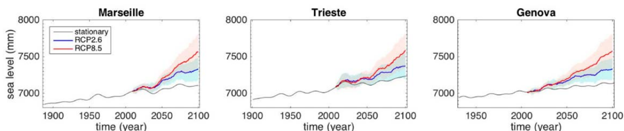
FIGURA 14-2. PREVISIONI MINIME E MASSIME DELL'INNALZAMENTO DEL MARE A MARSIGLIA, TRIESTE E GENOVA (DA VECCHIO ET AL. 2019)
