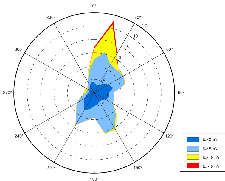
FIGURA 5-6. DIAGRAMMA DI DISTRIBUZIONE DIREZIONALE DEI VENTI OSSERVATI ALLA STAZIONE MAREOGRAFICA RMN DI GENOVA (GEN.1999 - NOV. 2019)
