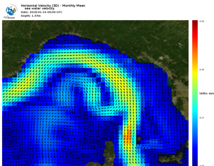
FIGURA 13-2. VALORE MEDIO DELLA CORRENTE SUPERFICIALE RICOSTRUITA PER IL MESE DI GENNAIO 2018.
