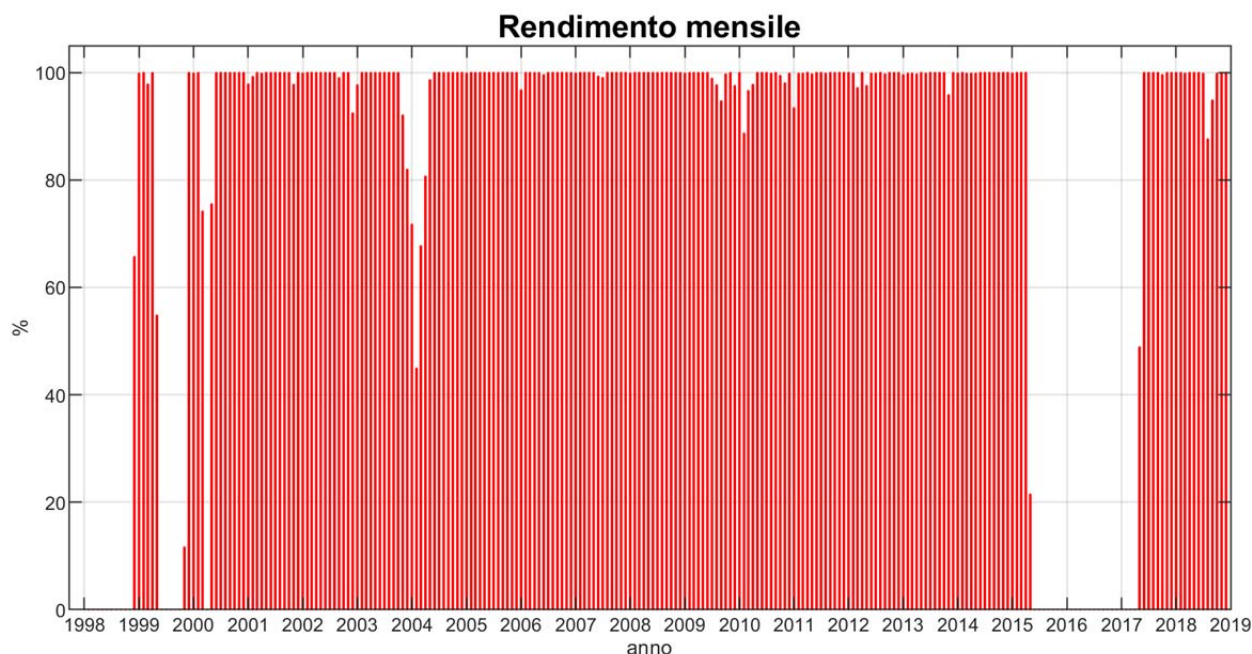
FIGURA 12-1. RENDIMENTI MENSILI DELLA STAZIONE MAREOGRAFICA RMN DI GENOVA. PERIODO DI RIFERIMENTO DICEMBRE 1998 - DICEMBRE 2019.
