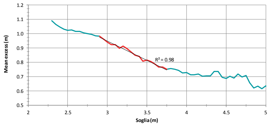
FIGURA 8-4 - MEAN RESIDUAL LIFE PLOT - SETTORE B: 105 - 180°N
