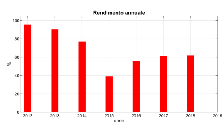
FIGURA 6-7. RENDIMENTO ANNUALE DELLA BOA ONDAMETRICA DI CAPO MELE FEBBRAIO 2012 - DICEMBRE 2018.
