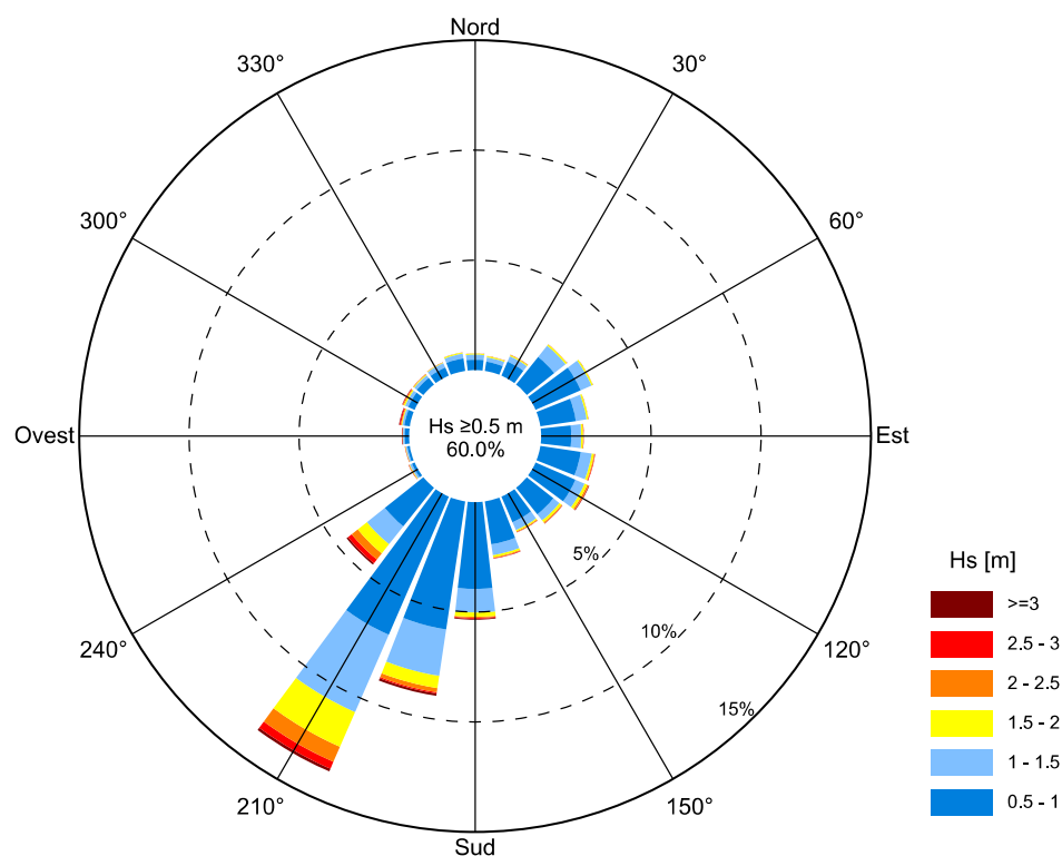
FIGURA 6-9. DISTRIBUZIONE DIREZIONALE DELL'ALTEZZA D'ONDA SIGNIFICATIVA H_s REGISTRATA DALLA BOA ONDAMETRICA DI CAPO MELE. PERIODO DI RIFERIMENTO FEBBRAIO 2012 - SETTEMBRE 2019
