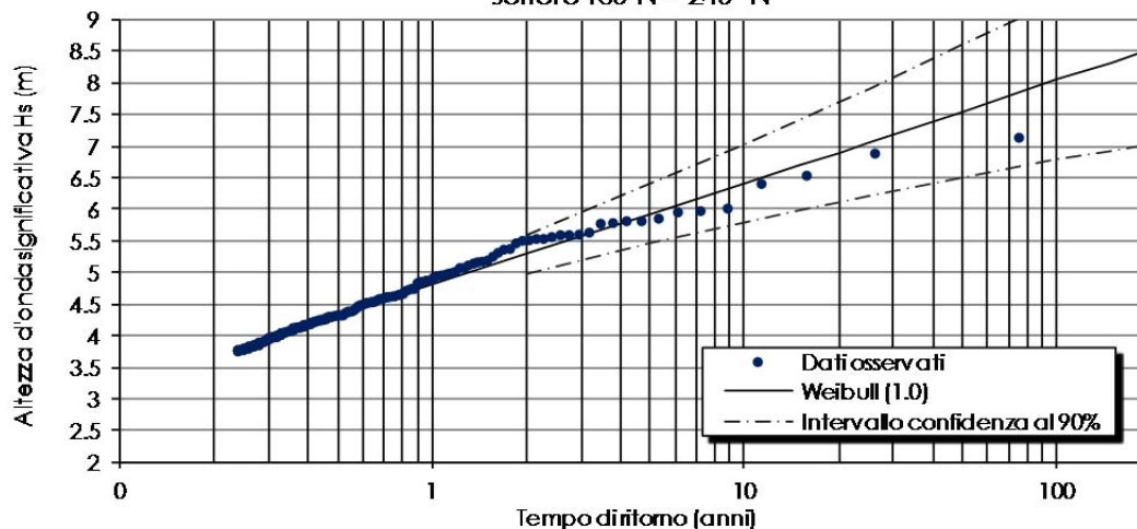
FIGURA 8-6 - GENOVA LARGO – SETTORE A: 180 - 240°N. VALORI DELL'ALTEZZA D'ONDA SIGNIFICATIVA IN FUNZIONE DEL TEMPO DI RITORNO SECONDO LE DIVERSE DISTRIBUZIONI STATISTICHE - METODO P.O.T. (PERIODO:1 GENNAIO 1979 - 31 DICEMBRE 2018)
