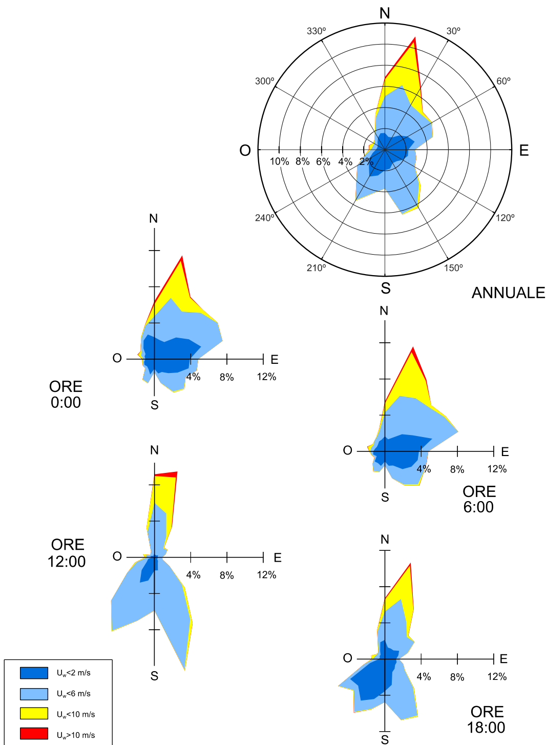
FIGURA 5-7. DISTRIBUZIONE DIREZIONALE DEI VENTI REGISTRATI DALLA STAZIONE RMN DI GENOVA SU BASE ORARIA 0:00, 6:00, 12:00, 18:00 (UTC) (PERIODO DI RIFERIMENTO 1999-2019).
