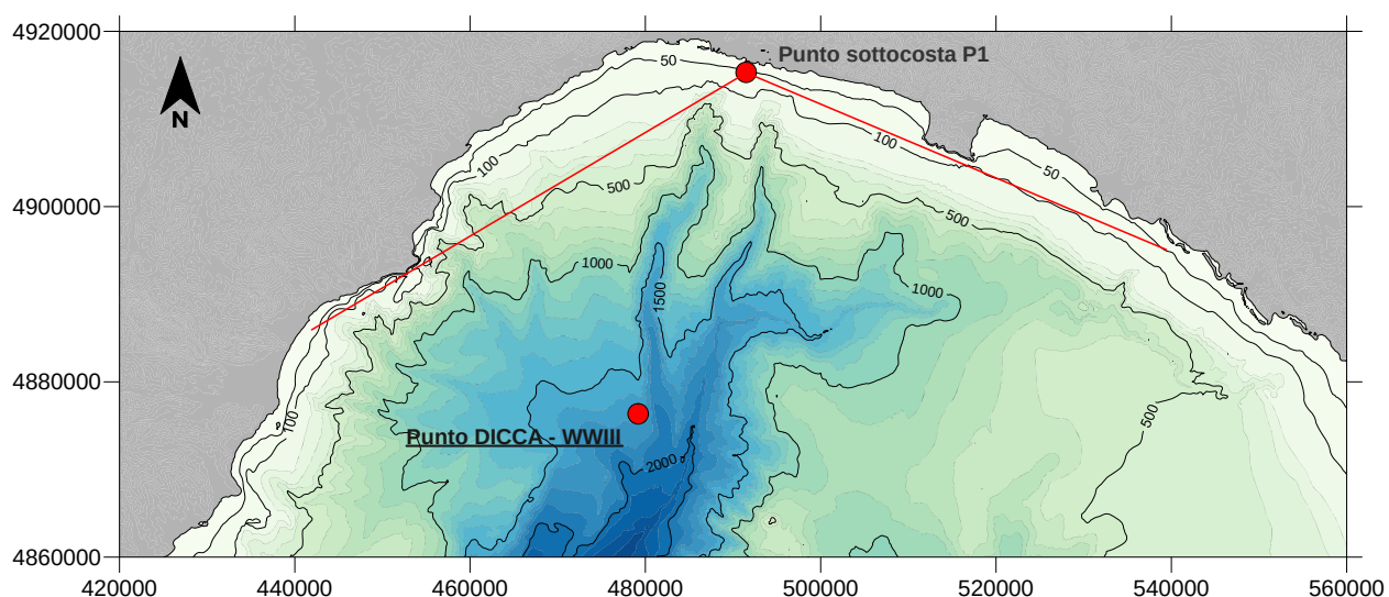
FIGURA 10-1. GRIGLIA DI CALCOLO UTILIZZATA PER LA MODELLAZIONE DELLA PROPAGAZIONE DEL MOTO ONDOSO CON I MODELLI MEROPE E SWAN ED INDICAZIONE DELLA POSIZIONE DEL PUNTO P1 ALL'ESTERNO DEL PORTO DI GENOVA.
