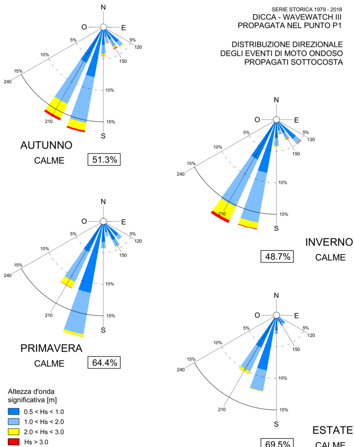
FIGURA 10-4. DISTRIBUZIONE DIREZIONALE DEGLI EVENTI DI MOTO ONDOSO PROPAGATI SOTTOCOSTA NEL PUNTO P1 CON IL MODELLO DI INVERSA SPETTRALE SU BASE STAGIONALE.
