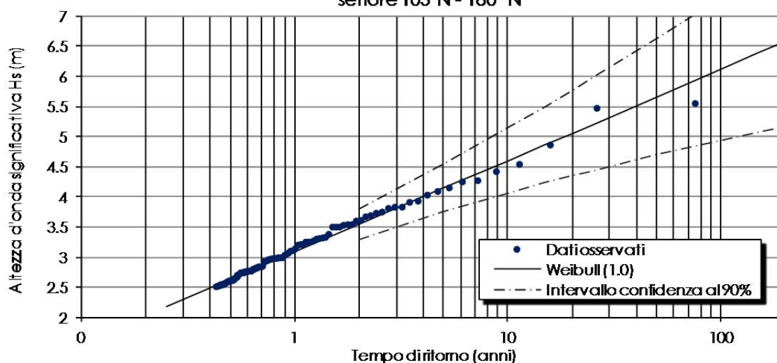
FIGURA 8-7 - GENOVA LARGO – SETTORE A: 105 -180°N. VALORI DELL'ALTEZZA D'ONDA SIGNIFICATIVA IN FUNZIONE DEL TEMPO DI RITORNO SECONDO LE DIVERSE DISTRIBUZIONI STATISTICHE - METODO P.O.T. (PERIODO:1 GENNAIO 1979 - 31 DICEMBRE 2018)
