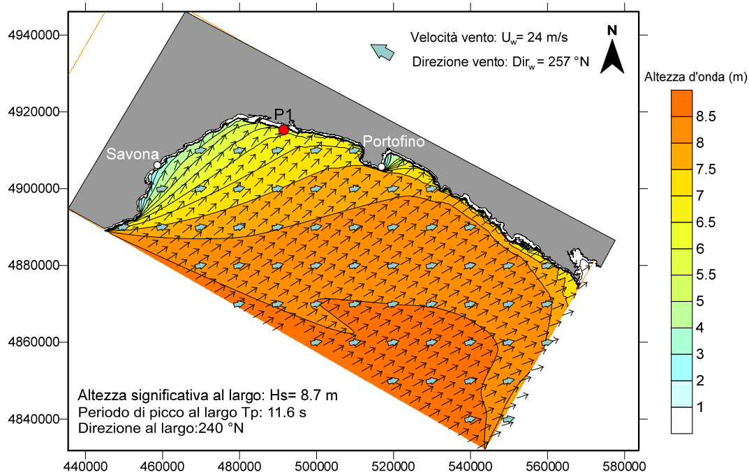
FIGURA 11-7 - RISULTATO DELLA PROPAGAZIONE DELLO STATO DI MARE OTTENUTO CON IL MODELLO SWAN. T_R=250 ANNI – DIREZIONE AL LARGO 240^\circ N
