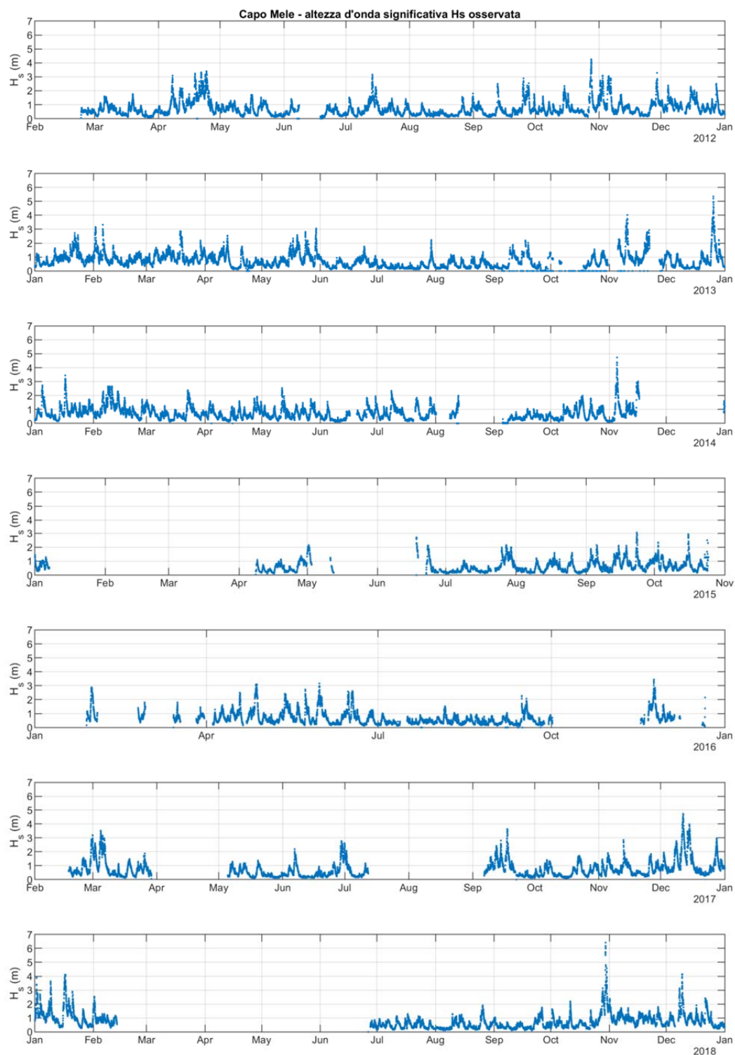
FIGURA 6-6. ALTEZZA D'ONDA SIGNIFICATIVA H_s MISURATA DALLA STAZIONE ONDAMETRICA DI CAPO MELE (PERIODO FEBBRAIO 2012 - DICEMBRE 2018).
