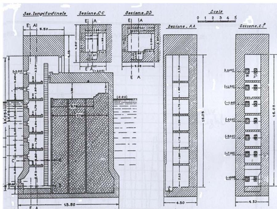
FIGURA 4-1. SEZIONI DEL CASSONE SPECIALE COSTRUITO PER IL RILEVAMENTO DELLA PRESSIONE ESERCITATA DALL'ONDA SULLA PARETE VERTICALE FINO A QUOTA -10.00.
