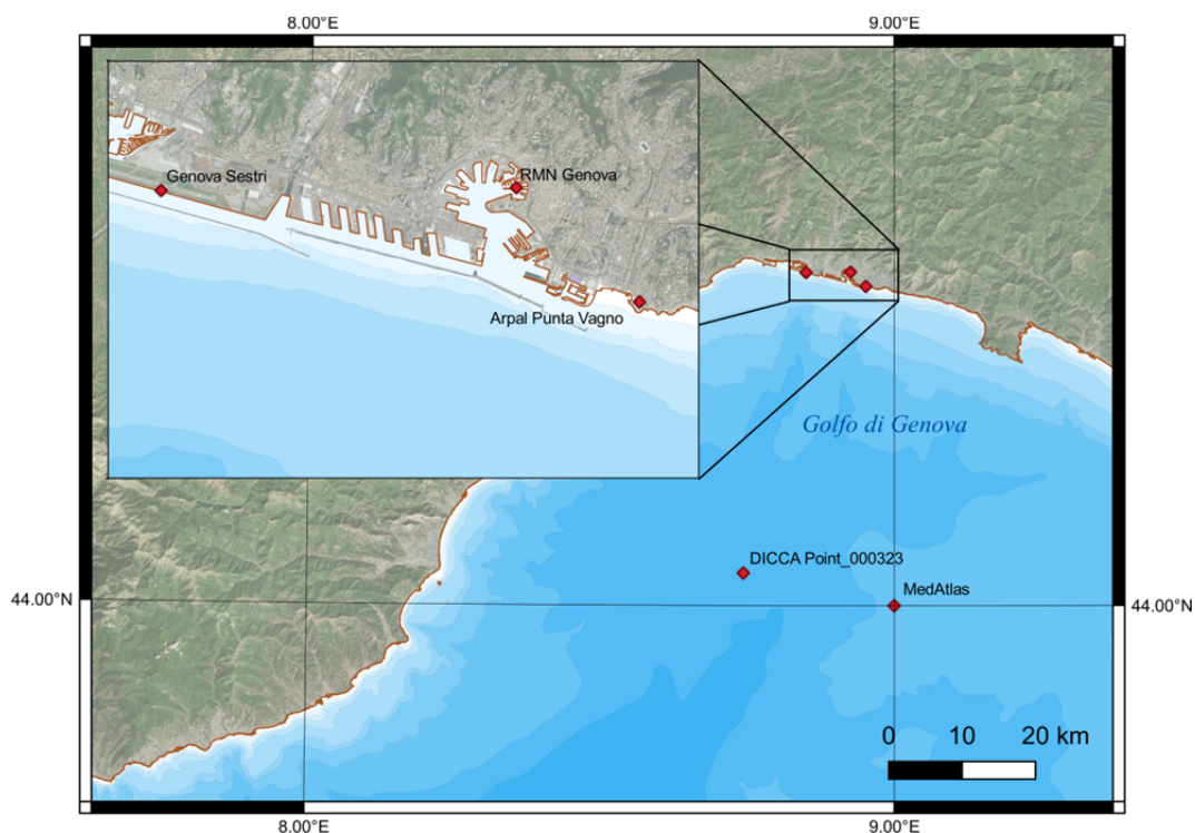
FIGURA 5-1. LOCALIZZAZIONE DELLE DIVERSE FONTI DI DATI ANEMOMETRICI UTILIZZATE PER LA DEFINIZIONE DEL REGIME DEI VENTI AL LARGO E SOTTOCOSTA.
