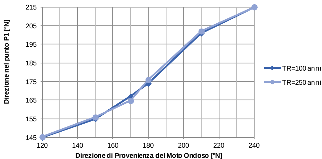
FIGURA 11-13 – DIREZIONE DEL MOTO ONDOSO OTTENUTA NEL PUNTO P1 IN FUNZIONE DELLA DIREZIONE DI PROVENIENZA AL LARGO PER GLI STATI DI MARE ESTREMI CON TEMPO DI RITORNO TR 100 ANNI E TR 250 ANNI..
