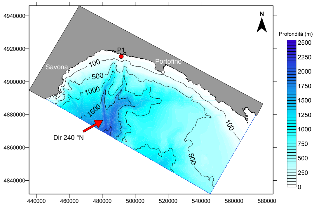
FIGURA 11-1. GRIGLIE DI CALCOLO UTILIZZATE PER LE SIMULAZIONI CONDOTTE CON IL MODELLO NUMERICO SWAN
