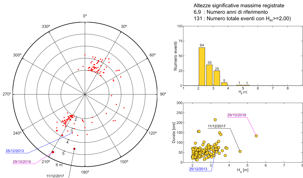
FIGURA 6-16. DISTRIBUZIONE DELLE ALTEZZE D'ONDA AL COLMO DELLE MAREGGIATE RICOSTRUITE AL LARGO DI CAPO MELE NEL PUNTO DICCA 000354 PERIODO FEB. 2012 - DIC. 2018
