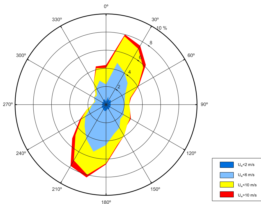
FIGURA 5-4. DISTRIBUZIONE DEI VENTI FORNITI DAL MEDATLAS AL LARGO DI GENOVA. COORDINATE 44^\circ\text{N}-9^\circ\text{E} . PERIODO DI RIFERIMENTO 1992-2001.
