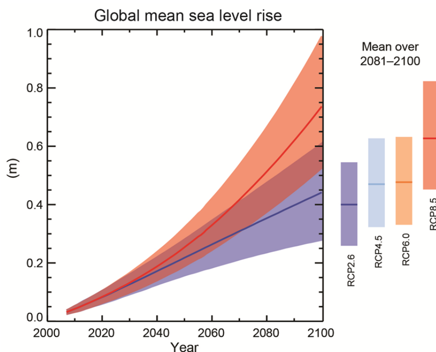
FIGURA 14-1. PREVISIONE PER IL GLOBAL SEA LEVEL RISE FORNITA DALL'IPCC.
