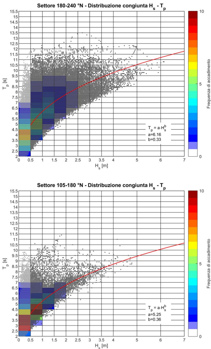
FIGURA 9-6. DISTRIBUZIONE CONGIUNTA DEI VALORI H_s E T_p E LEGGE DI ADATTAMENTO PER I DATI DI MOTO ONDOSO RICOSTRUITI DAL DICCA AL LARGO DI GENOVA. IN ALTO SETTORE DI TRAVERSA PRINCIPALE (180 - 240 °N). IN BASSO SETTORE DI TRAVERSA SECONDARIO (105 - 180°N)
