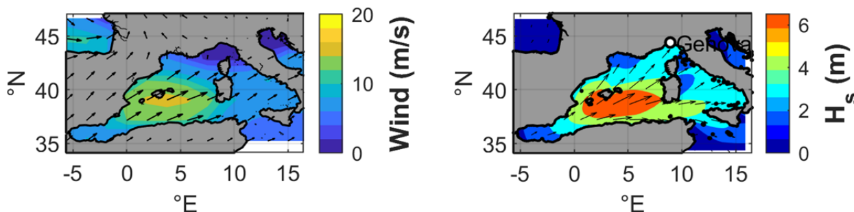
FIGURA A-3. CAMPI DI VENTO E DI ALTEZZA D'ONDA SIGNIFICATIVA H_s OTTENUTI A SEGUITO DELLA SIMULAZIONE CON IL MODELLO SWAN PER IL GIORNO 18 FEBBRAIO 1955
