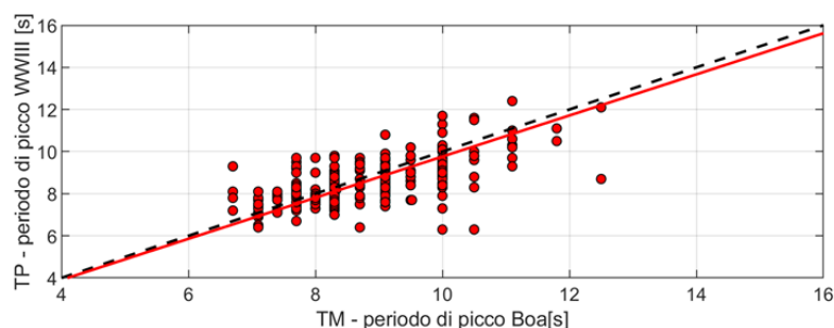
FIGURA 7-4. CONFRONTO ASINCRONO TRA I VALORI DI PERIODO DI PICCO T_p AL COLMO DELLE MAREGGIATE (CON H_s > 3.0 m) REGISTRATI DALLA BOA RON DI LA SPEZIA TRA IL 1989 ED IL 2014 E QUELLI RICOSTRUITI DAL DICCA CON IL MODELLO WWIII
