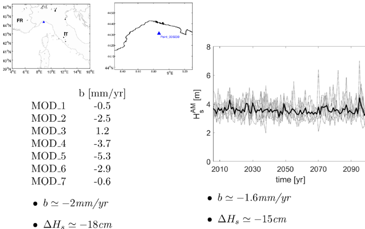
FIGURA 14-3. STIMA DELLA VARIAZIONE DI H_s AL 2100 DOVUTA AI POSSIBILI CAMBIAMENTI CLIMATICI IN UN PUNTO AL LARGO DI GENOVA EFFETTUATA DAL DICCA DI GENOVA. (FONTE: TRENDS AND VARIABILITY OF WAVES UNDER SCENARIO RCP8.5 IN THE MEDITERRANEAN SEA - G.BESIO, L.MENTASCHI, F. DE LEO - 12 nd INTERNATIONAL WORKSHOP ON WAVES, STORM SURGES AND COASTAL HAZARDS)
