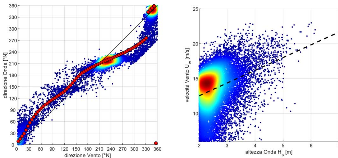
FIGURA 9-1. STATI DI MOTO ONDOSO CON H_s > 2.0 m E U_w > 6.0 m/s APPARTENENTI ALLA SERIE STORICA DICCA AL LARGO DEL GOLFO DI GENOVA (1979-2018).
