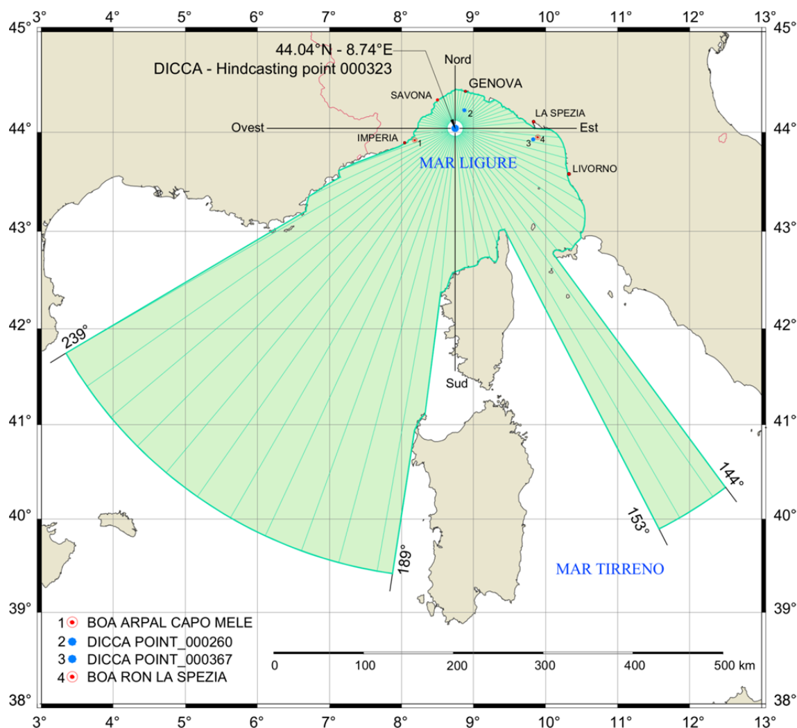
FIGURA 2-4. FETCH GEOGRAFICO AL LARGO DEL GOLFO DI GENOVA PUNTO DI COORDINATE 44.04°N - 8.74°E.
