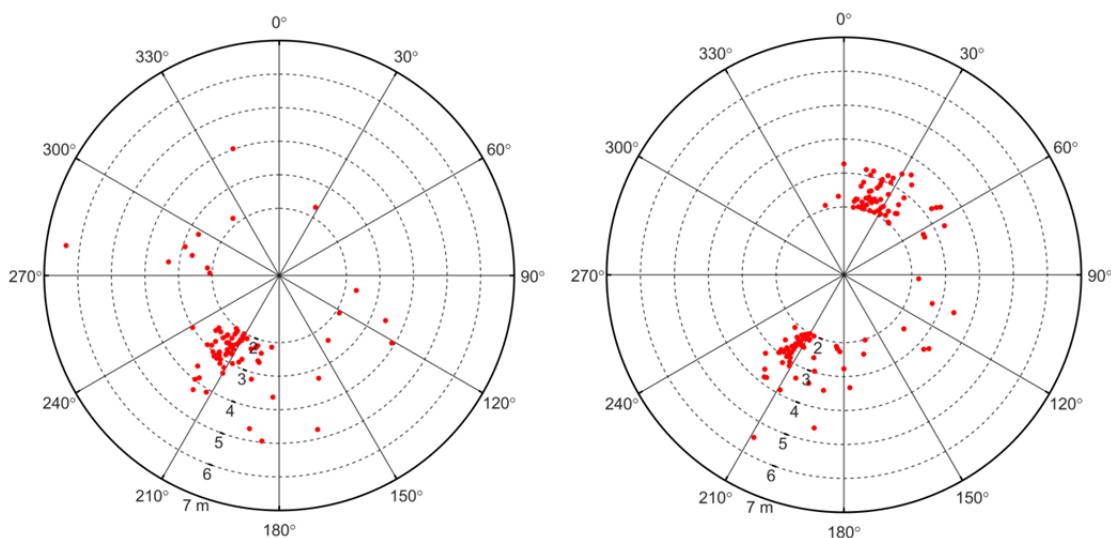
FIGURA 7-5. DISTRIBUZIONE DEI VALORI DI ALTEZZA D'ONDA H_s AL COLMO DELLE MAREGGIATE REGISTRATE DALLA BOA ARPAL DI CAPO MELE (SINISTRA) E RICOSTRUITE DAL DICCA (DESTRA) NEL PERIODO 2012 - 2018.
