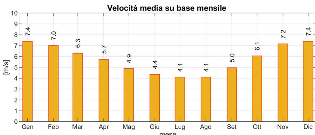
FIGURA 5-3. VELOCITÀ MEDIA SU BASE MENSILE DEI VENTI IN RICOSTRUZIONE FORNITI DAL DICCA AL LARGO DEL GOLFO DI GENOVA NEL PUNTO 000323 (PERIODO DI RIFERIMENTO 1979-2018)
