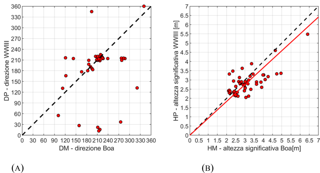
FIGURA 7-6. CONFRONTO ASINCRONO TRA I VALORI AL COLMO DELLE MAREGGIATE (CON H_s > 2.0 M) REGISTRATI DALLA BOA ARPAL DI CAPO MELE TRA IL 2012 ED IL 2018 E QUELLI RICOSTRUITI DAL DICCA CON IL MODELLO WWIII IN PROSSIMITÀ DELLA BOA. (A) CORRELAZIONE DIREZIONE BOA/DIREZIONE WWIII (B) CORRELAZIONE H_s BOA/ H_s WWIII.
