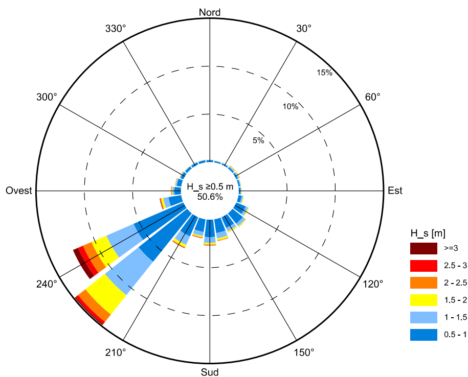
FIGURA 6-18. DISTRIBUZIONE DIREZIONALE DELL'ALTEZZA D'ONDA SIGNIFICATIVA H_s RICOSTRUITA DAL DICCA NEL PUNTO P_000367 AL LARGO DI LA SPEZIA - PERIODO DI RIFERIMENTO 1979-2018
