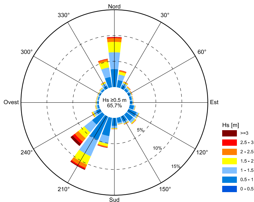
FIGURA 6-12. DISTRIBUZIONE DIREZIONALE DELL'ALTEZZA D'ONDA SIGNIFICATIVA H_s RICOSTRUITA DAL DICCA NEL PUNTO P_000323 AL LARGO DEL GOLFO DI GENOVA - PERIODO DI RIFERIMENTO 1979-2018.
