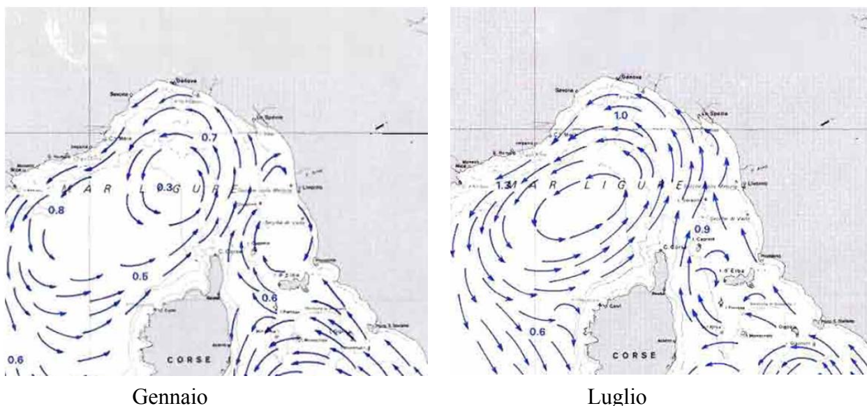
FIGURA 13-1. CARTE DELLE CORRENTI SUPERFICIALI PER I MESI DI GENNAIO E LUGLIO. ESTRATTE DALLA PUBBLICAZIONE 3068 "ATLANTE DELLE CORRENTI SUPERFICIALI DEI MARI D'ITALIA" REDATTA DALL'ISTITUTO IDROGRAFICO DELLA MARINA ITALIANA.
