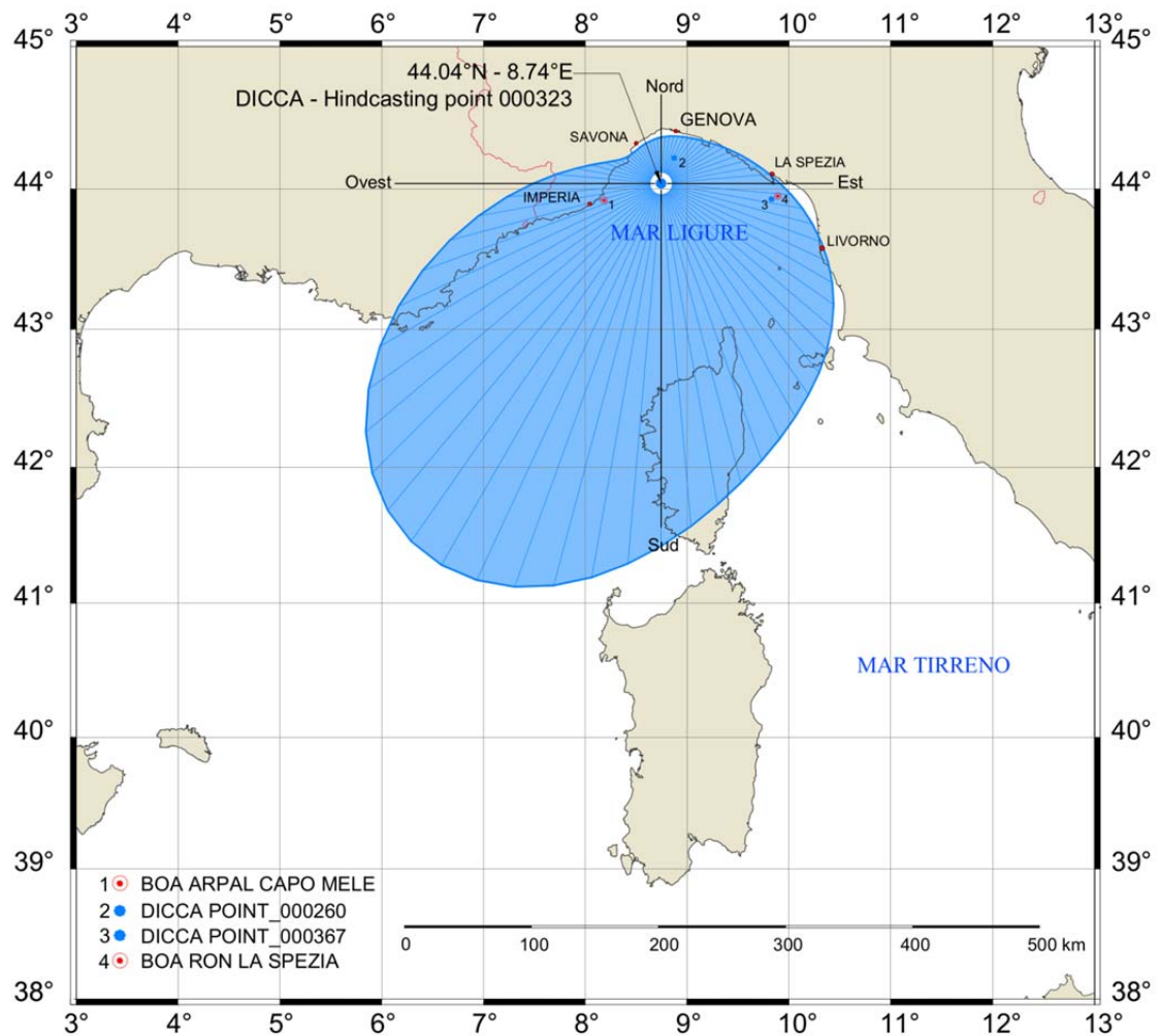
FIGURA 2-5. FETCH EFFICACE AL LARGO DEL GOLFO DI GENOVA PUNTO DI COORDINATE 44.04°N - 8.74°E.
