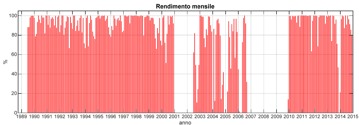
FIGURA 6-3. RENDIMENTO MENSILE DELLA BOA ONDAMETRICA RON DI LA SPEZIA LUGLIO 1989 - DICEMBRE 2014.
