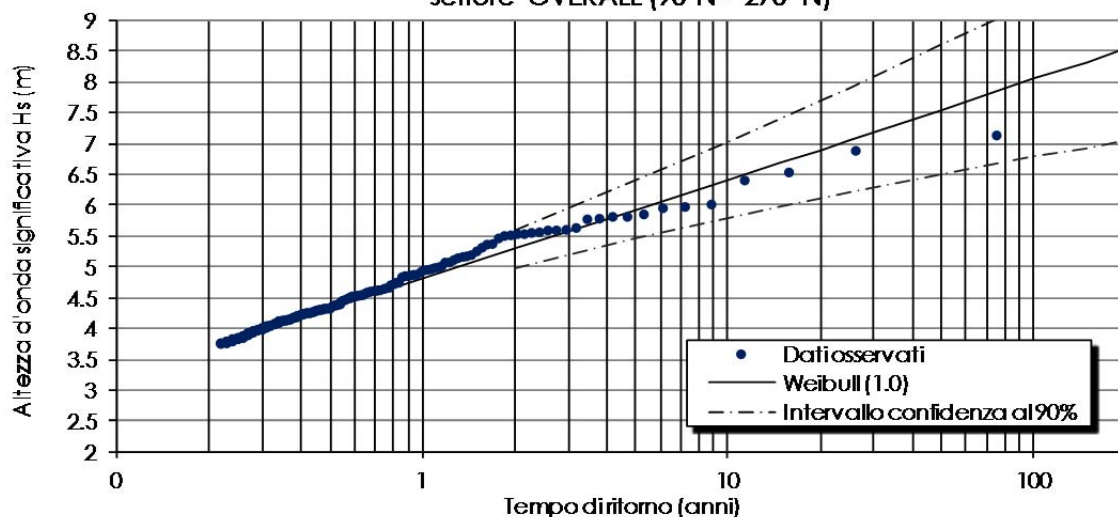
FIGURA 8-8 - GENOVA LARGO – SETTORE OVERALL: 90-270°N. VALORI DI H s IN FUNZIONE DEL TEMPO DI RITORNO PER LE DIVERSE DISTRIBUZIONI STATISTICHE - METODO P.O.T. (PERIODO: 1979 - 2018)
